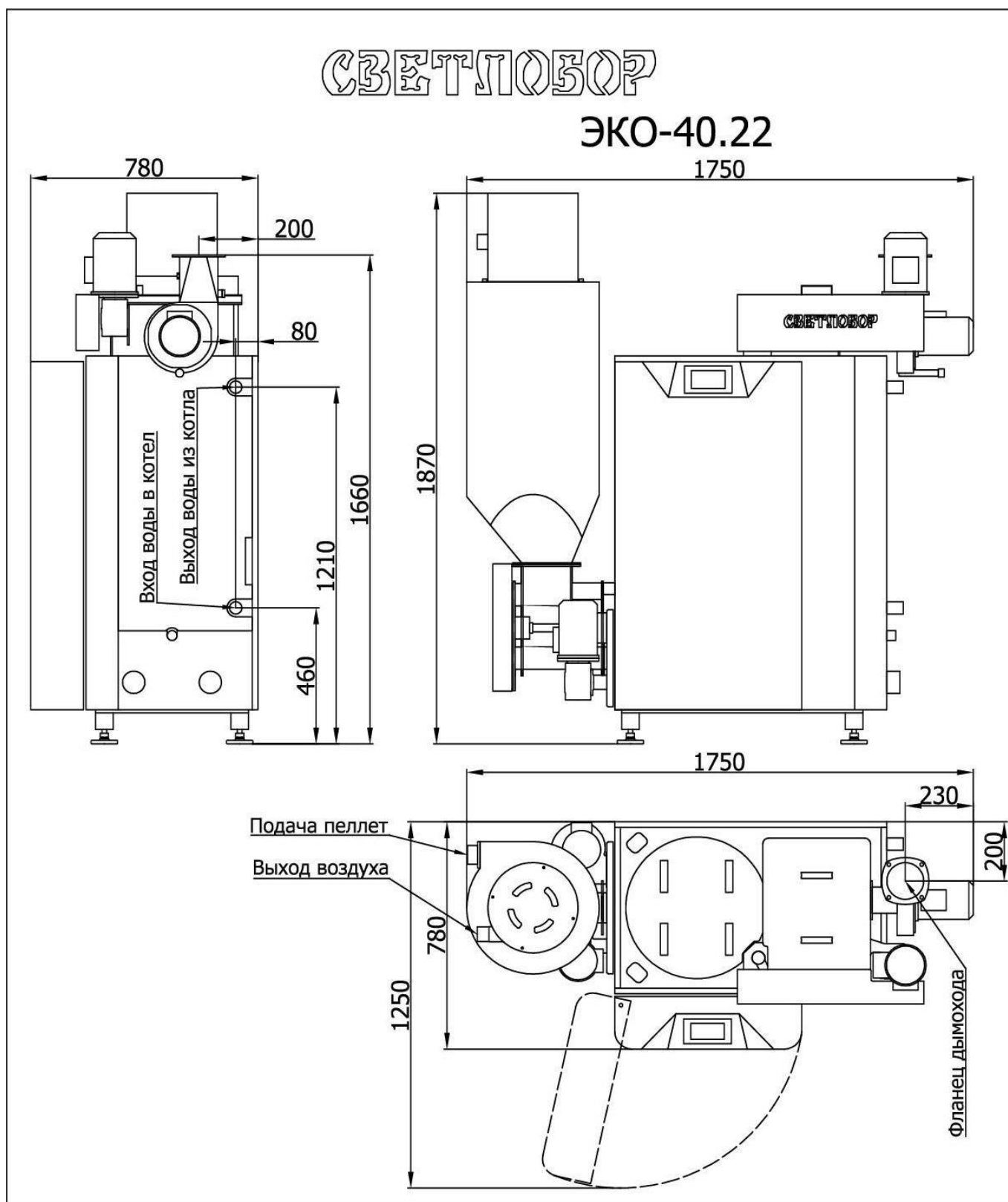
Рис. 1. Габаритные размеры
