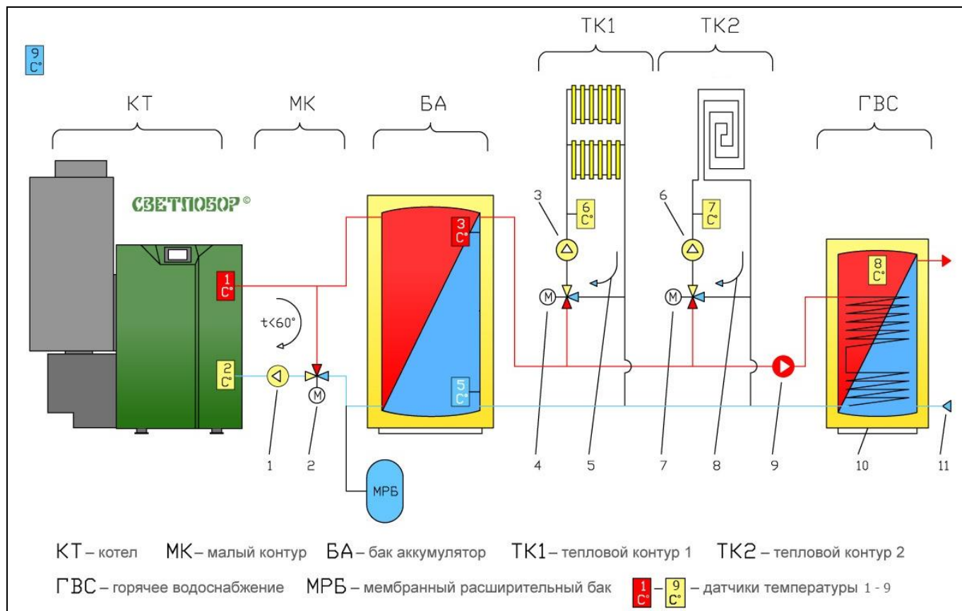
Принципиальная схема подключения
