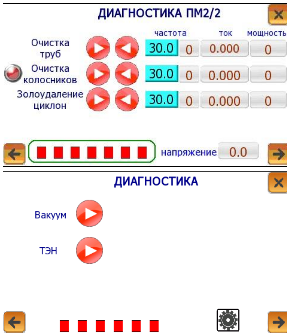
Включение отдельных агрегатов котла
