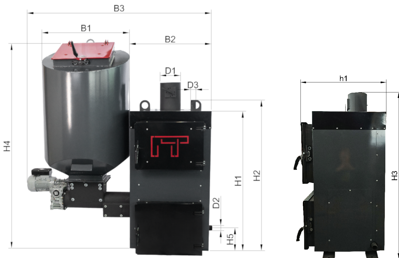
Рисунок 1. Габаритные размеры котлов, мощностью 10-20 кВт.
