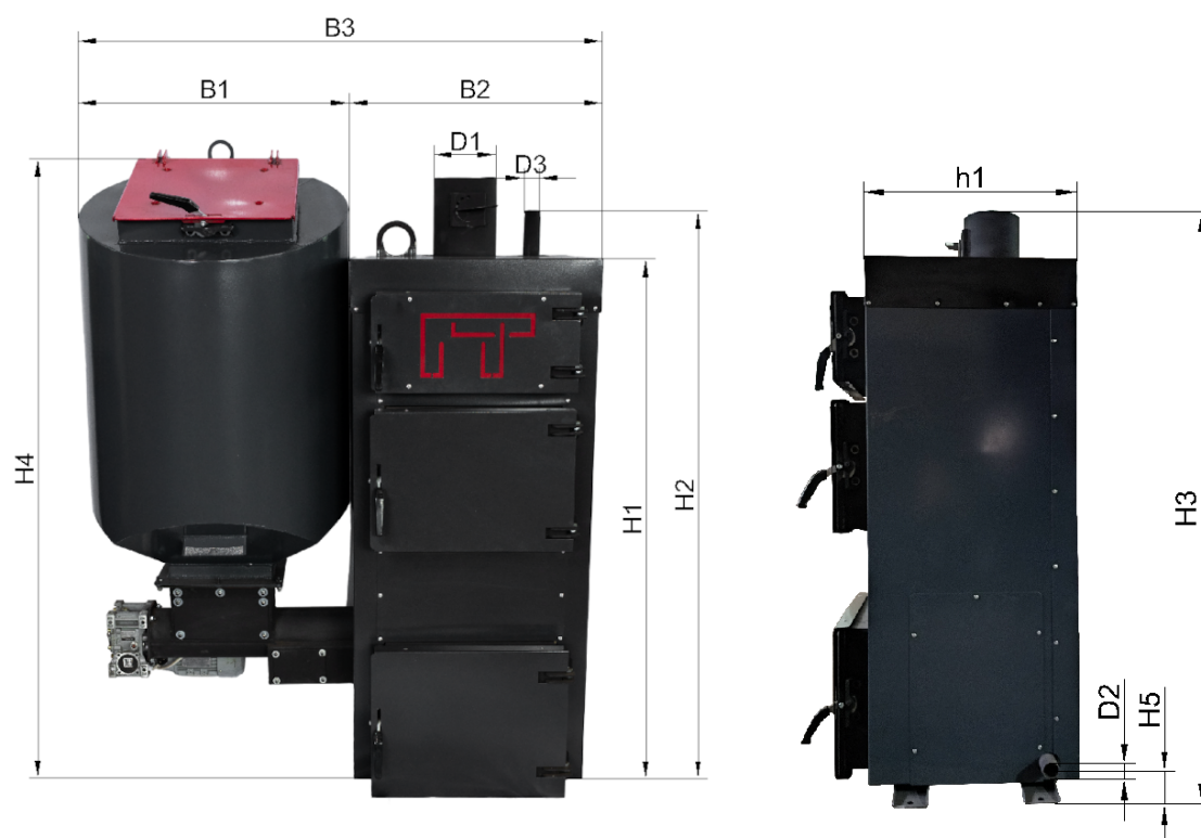
Рисунок 2. Габаритные размеры котлов, мощностью 25-80 кВт.
