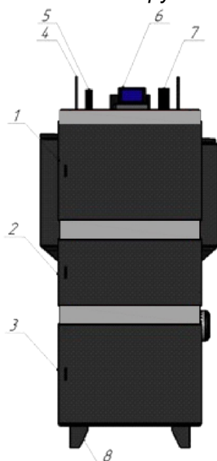
Рисунок 7 — Схема размещения составных элементов в котлах серии ПРОМ-ТЕПЛО(вид с фронта). 1-дверца теплообменника; 2-дверца горелки; 3-дверца зольника; 4-ухо транспортировочное; 5-группа безопасности; 6-контроллер; 7-труба подачи; 8-опора котла
