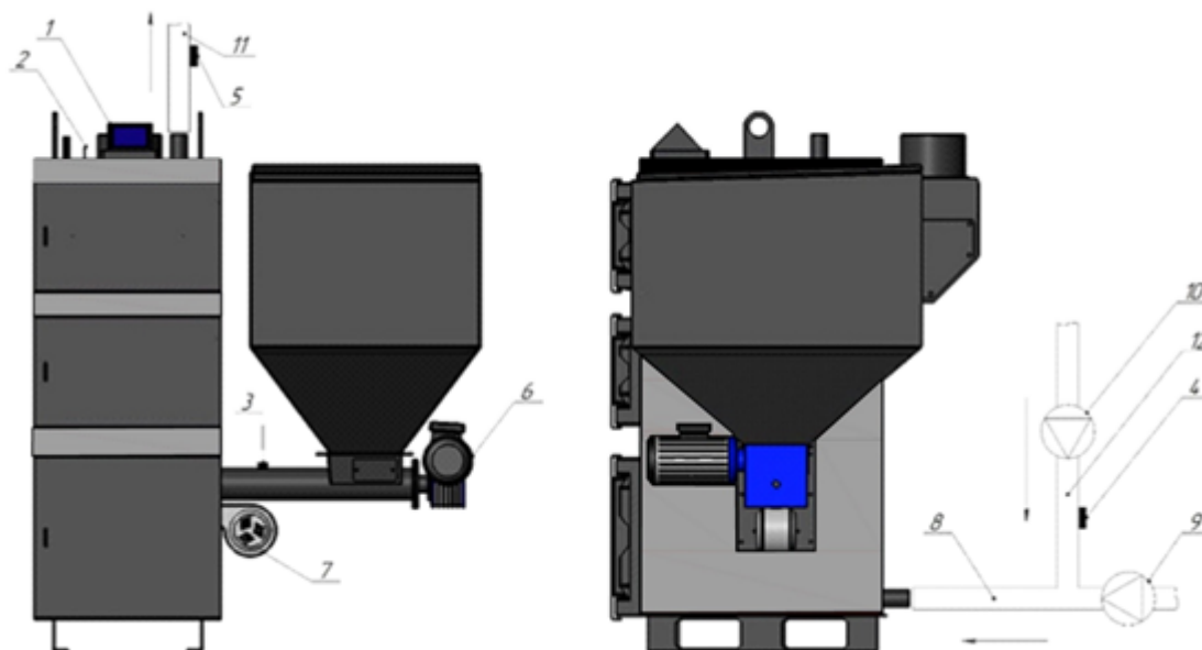
Рисунок 12 — Схема подключения блока управления к котлу. 1-контроллер (подключается к сети 220В); 2-датчик системы отопления (устанавливается в гильзу); 3-датчик шнека; 4-датчик горячего водоснабжения (ГВС); 5-аварийный датчик (термик); 6-мотор-редуктор; 7-вентилятор наддува; 8-труба обратной линии от отопления; 9-насос системы отопления; 10-насос ГВС; 11-труба подачи; 12-труба обратной линии от бойлера ГВС.
