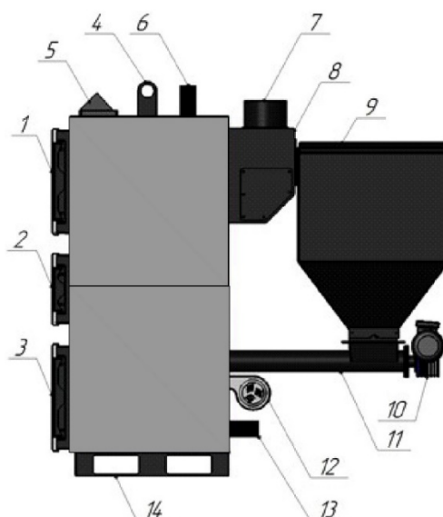
Рисунок 8 – Схема размещения составных элементов в котлах серии ПРОМ-ТЕПЛО(вид сбоку). 1-дверца теплообменника; 2-дверца горелки; 3-дверца зольника;; 4-ухо транспортировочное; 5-контроллер; 6-труба подачи; 7-дымовая труба; 8-короб дымохода; 9-бункер; 10-мотор-редуктор; 11-труба топливоподачи; 12-вентилятор наддува; 13-труба обратной линии; 14-опора котла.
