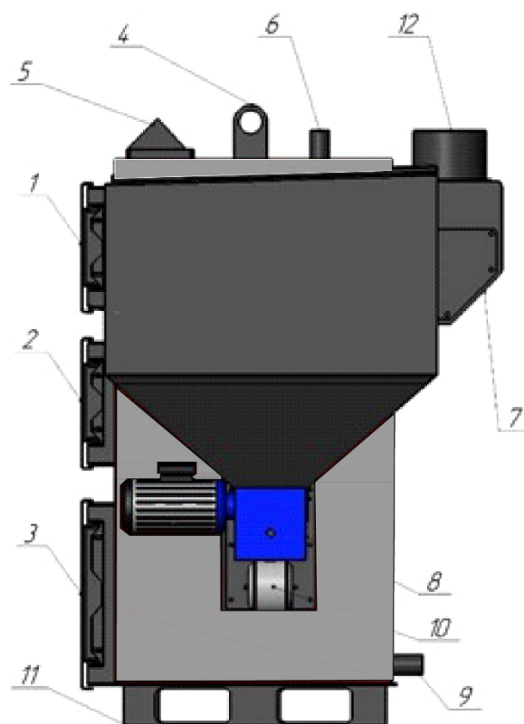
Рисунок 6 — Схема размещения составных элементов в котлах серии ПРОМ-ТЕПЛО(вид сбоку). 1-дверца теплообменника; 2-дверца горелки; 3-дверца зольника; 4-ухо транспортировочное; 5-контроллер; 6-труба подачи; 7-короб дымохода; 8-мотор-редуктор; 9-труба обратной линии; 10-вентилятор наддува; 11-опора котла; 12-дымовая труба.
