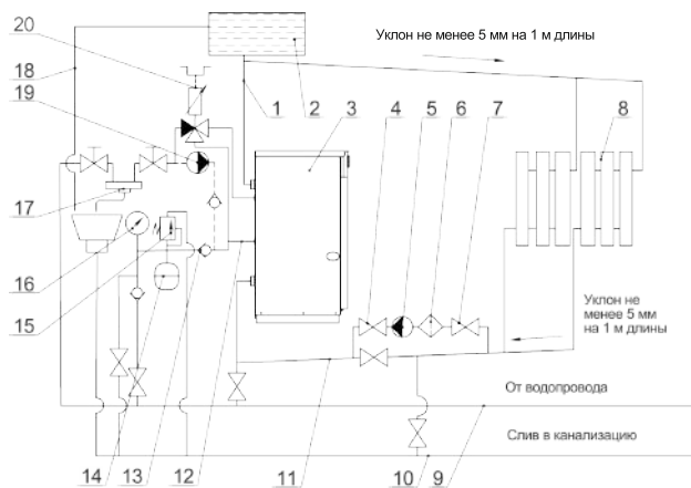
Рисунок 15 — Рекомендуемая гидравлическая схема системы отопления с циркуляционным насосом и схемой автоматического поддержания безопасной температуры ( \leq 60^\circ\text{C} ) в контуре горячего водоснабжения (ГВС) (с регулятором температуры).
