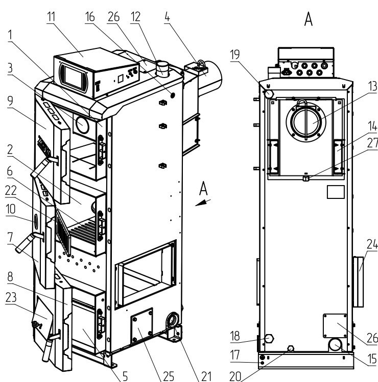
Рис.2 Котел отопительный.
