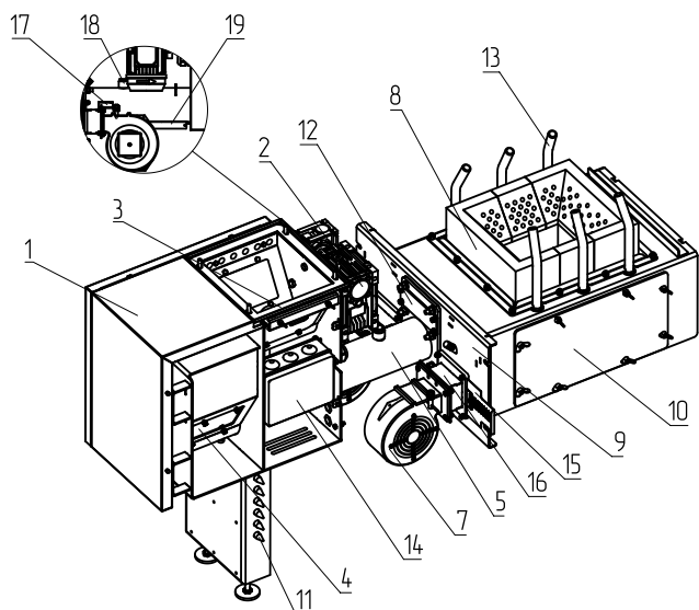
Рис.3.1 Горелка ретортная Stahano 85-135.
