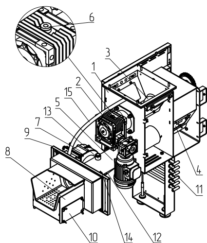
Рис.3 Горелка лотковая Stahano 16-65.
