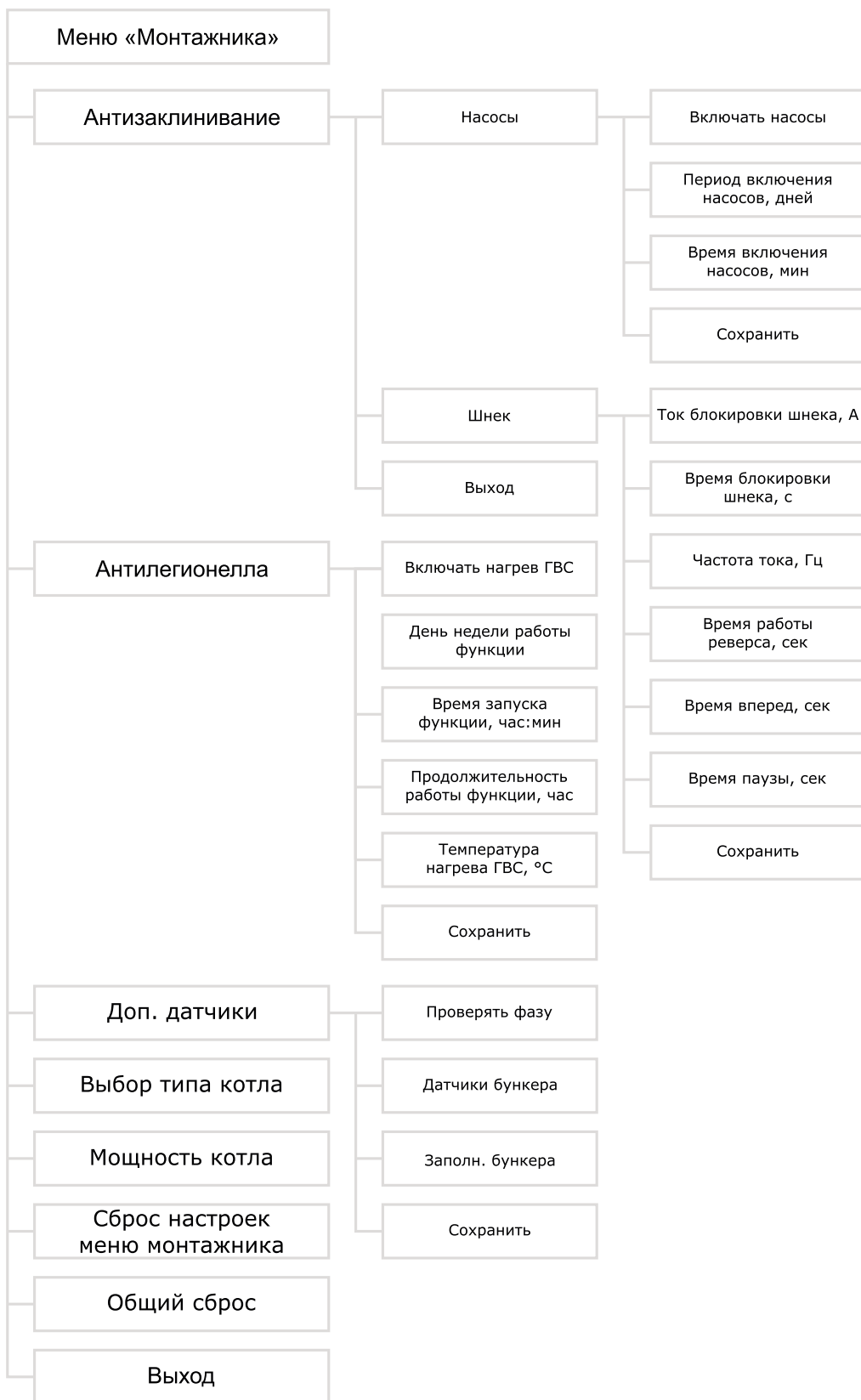
Рис.24 Блок-схема меню монтажника (продолжение)
