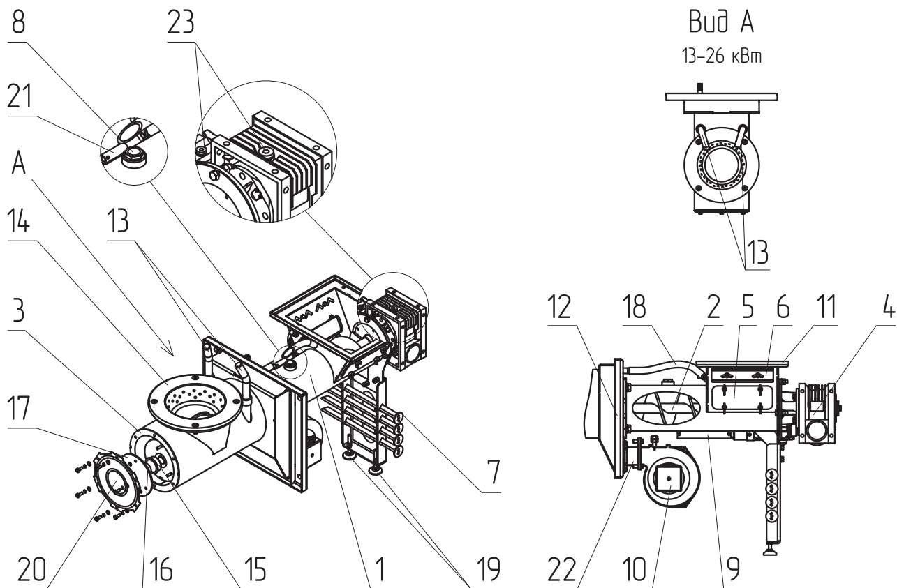
Рис.3 Механизм подачи топлива с горелкой котла
