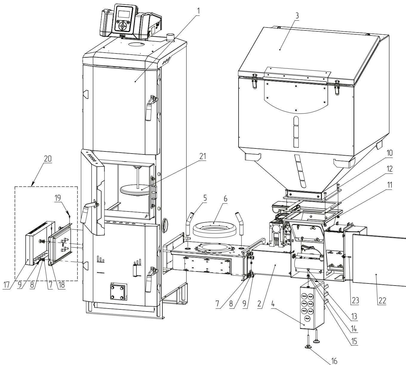
Рис.9 Монтаж котла
