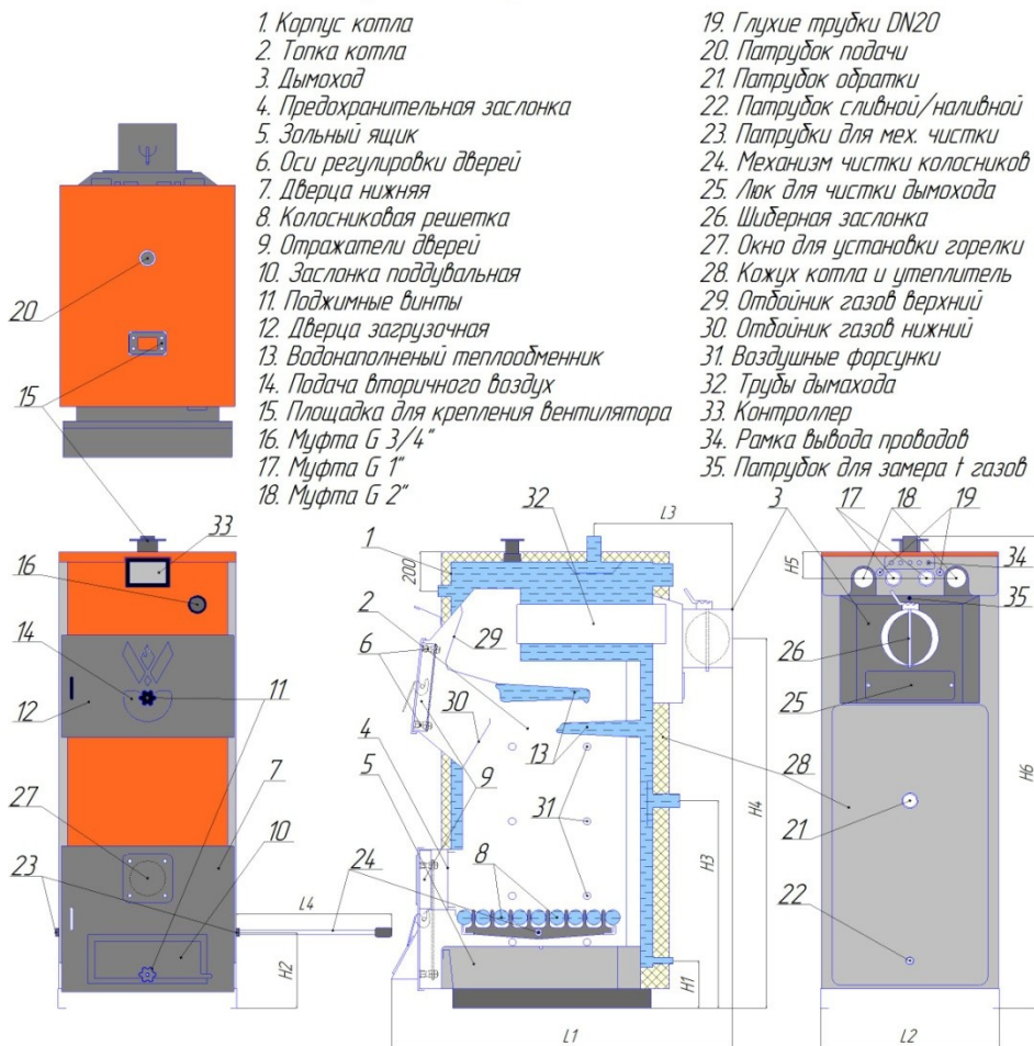
Рисунок 1. Устройство котлов WIRT Smart+
