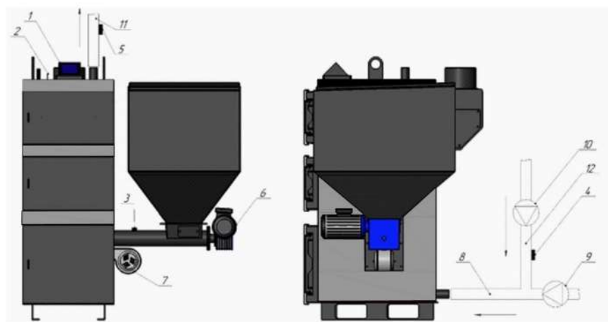
Рисунок 10 — Схема подключения блока управления к котлу. 1-контроллер (подключается к сети 220В); 2-датчик системы отопления (устанавливается в гильзу); 3-датчик шнека; 4-датчик горячего водоснабжения (ГВС); 5-аварийный датчик (термик); 6-мотор-редуктор; 7-вентилятор; 8-трубопровод обратной линии теплоносителя; 9-циркуляционный насос; 10-насос ГВС; 11-трубопровод подачи теплоносителя; 12-труба обратной линии от бойлера ГВС.
