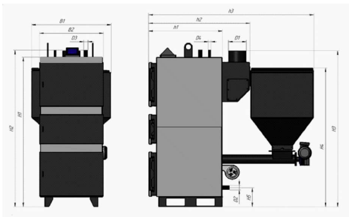
Рисунок 2. Габаритные размеры VULKAN BOSS, мощностью 330-470 кВт.
