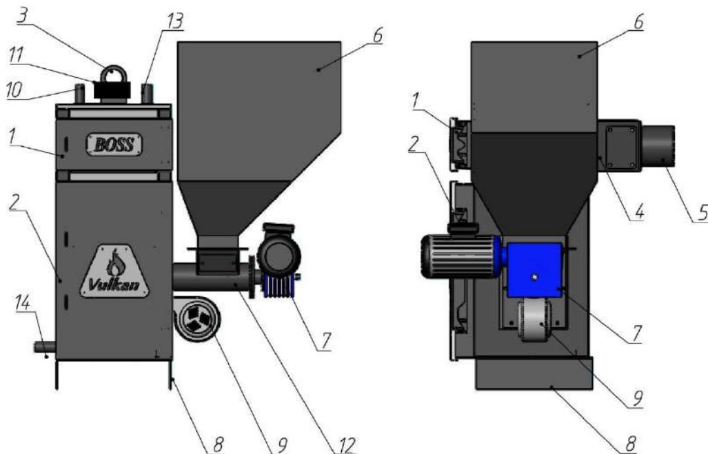
Рисунок 4. — Схема размещения составных элементов в котлах VULKAN серии BOSS. 1- дверца теплообменника; 2-дверца топочной камеры и зольника; 3-ухо транспортное; 4-короб дымохода; 5-труба дымовая; 6-бункер топлива; 7-мотор-редуктор; 8- опора котла; 9-вентилятор наддува; 10- патрубок под группу безопасности; 11-контроллер; 12-труба топливоподачи; 13-патрубок подачи теплоносителя; 14-патрубок обратной линии теплоносителя.
