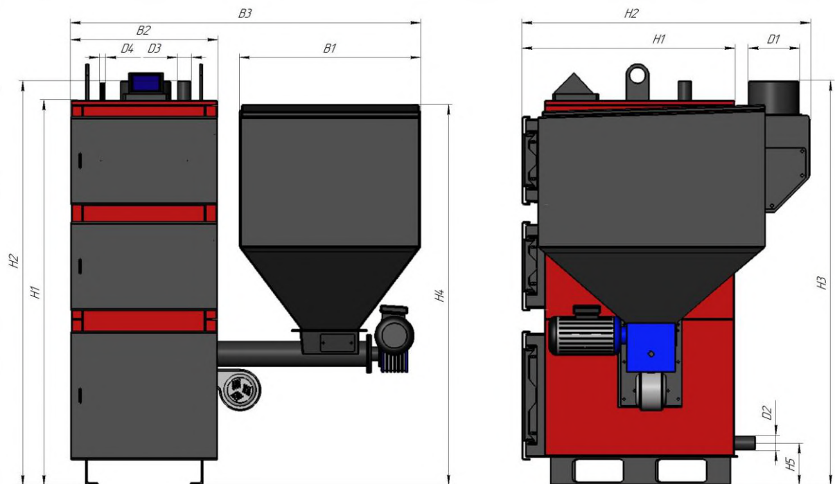
Схема для таблицы размеров VULKAN Еко, Еко Plus
