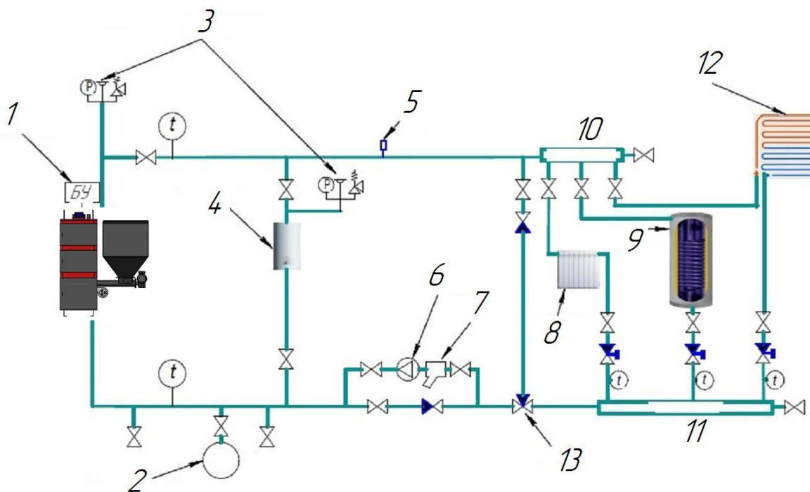
Рисунок 9 — Схема обвязки автоматического котла с трехходовым клапаном. 1-блок управления котлом; 2-расширительный бак; 3-группа безопасности; 4-электрокотел резервный; 5-воздухоотводчик; 6-насос циркуляционный; 7-фильтр; 8-радиатор; 9-бойлер; 10-коллектор подачи; 11-коллектор обратной подачи; 12-теплый пол; 13-клапан трехходовой.
