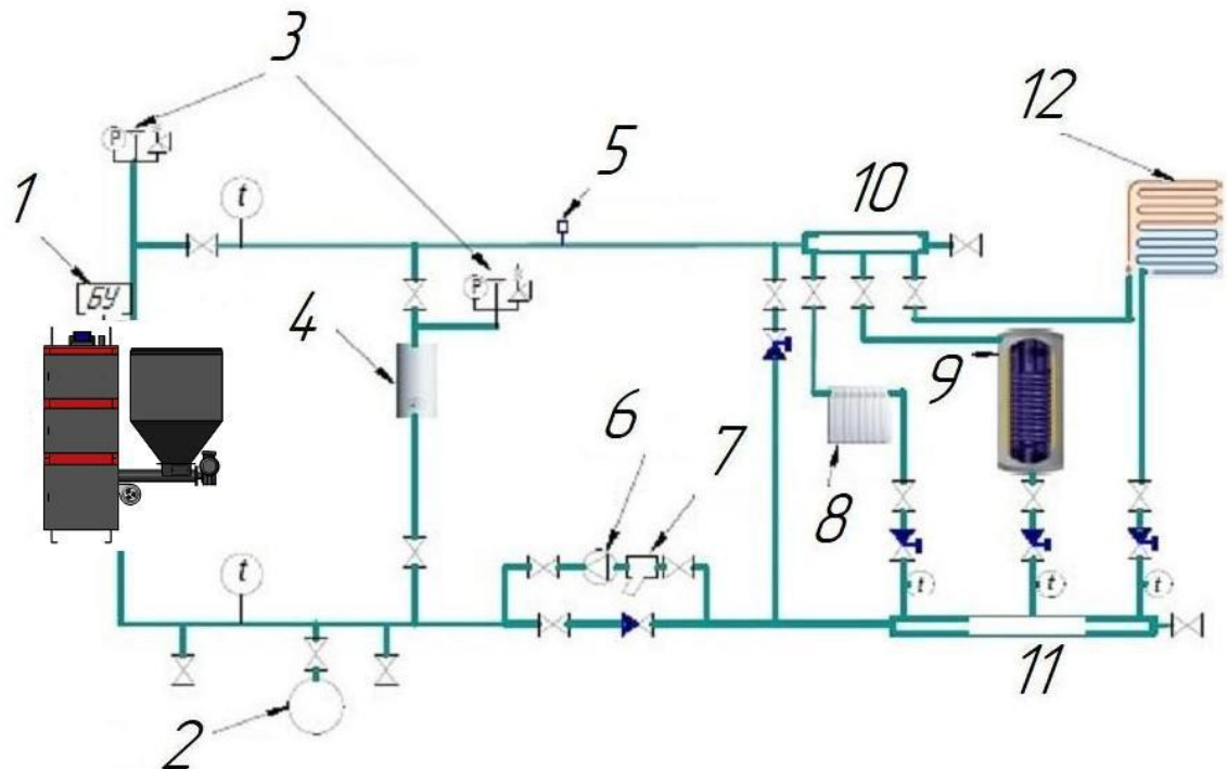
Рисунок 8 — Типовая схема обвязки автоматического котла. 1-блок управления котлом; 2-расширительный бак; 3-группа безопасности; 4-электродвигатель резервный; 5-воздухоотводчик; 6-насос циркуляционный; 7-фильтр; 8-радиатор; 9-бойлер; 10-коллектор подачи; 11-коллектор обратной подачи; 12-теплый пол
