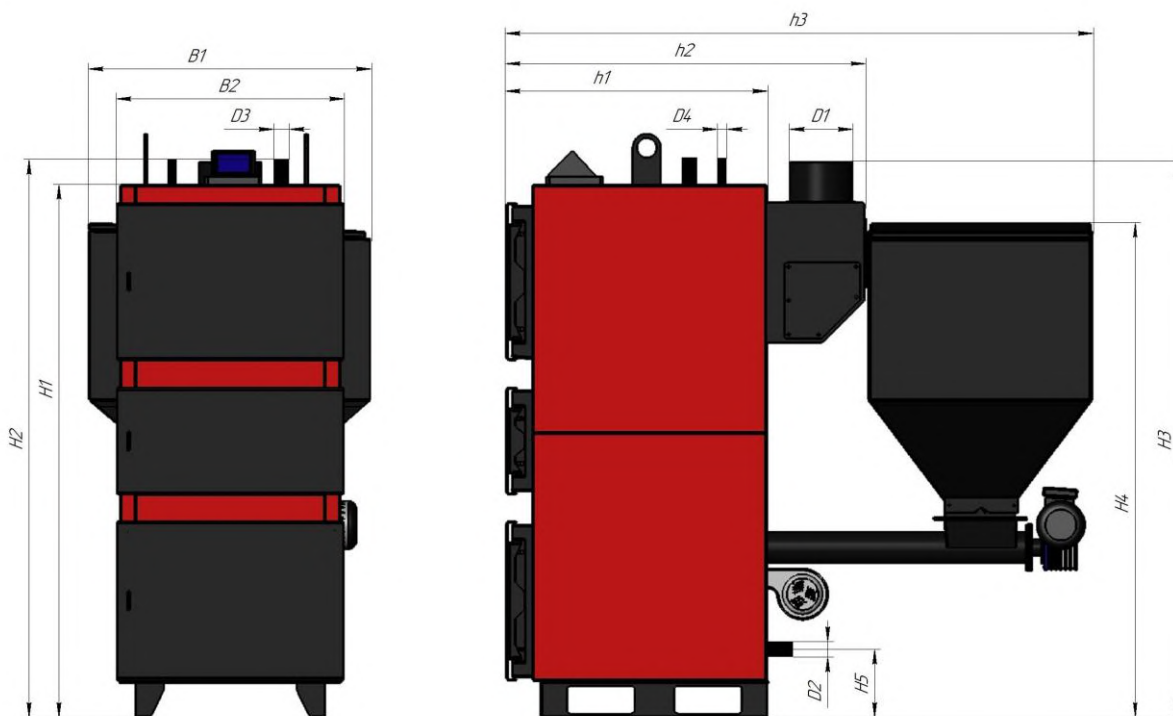
Схема для таблицы размеров VULKAN Еко-Z
