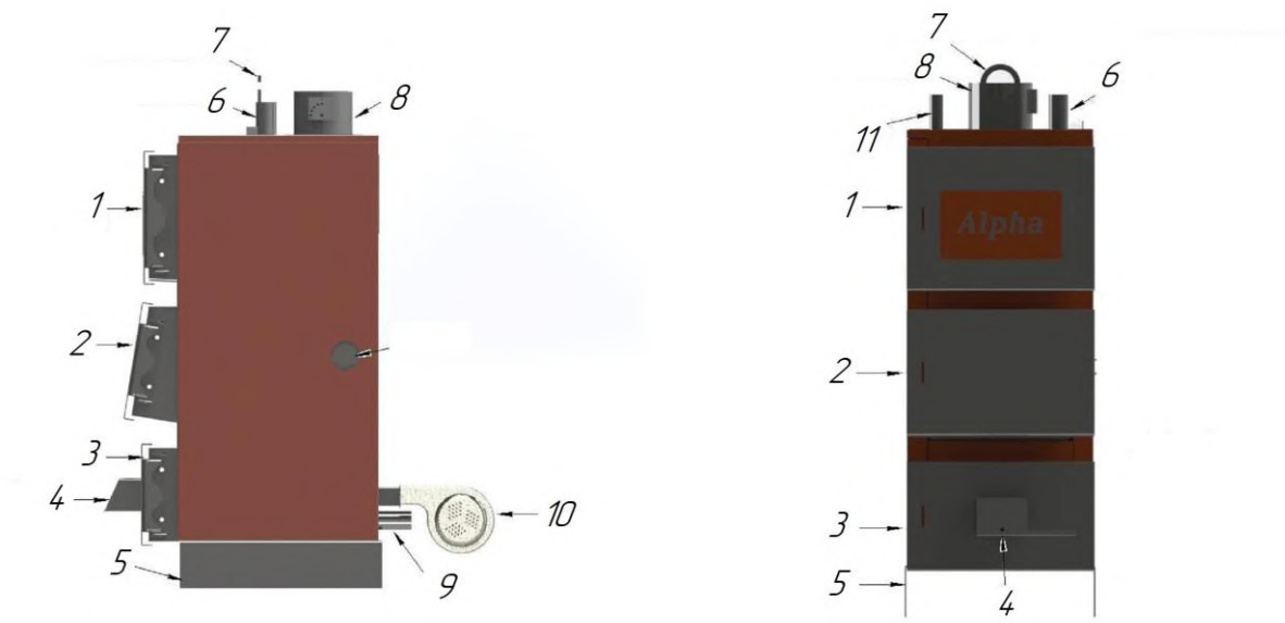
Рисунок 3 — Схема котла ALPHA. 1-дверь верхняя; 2-дверь средняя; 3-дверь нижняя; 4-окно поддува; 5-опора котла; 6-труба подачи; 7-ухо транспортировочное; 8-дымовая труба; 9-труба обратной линии; 10-вентилятор наддува; 11-патрубок группы безопасности
