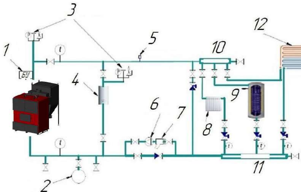
Рисунок 6 — Типовая схема обвязки автоматического котла. 1-блок управления котлом; 2-расширительный бак; 3-группа безопасности; 4-электродкотел резервный; 5-воздухоотводчик; 6-насос циркуляционный; 7-фильтр; 8-радиатор; 9-бойлер; 10-коллектор подачи; 11-коллектор обратной подачи; 12-теплый пол
