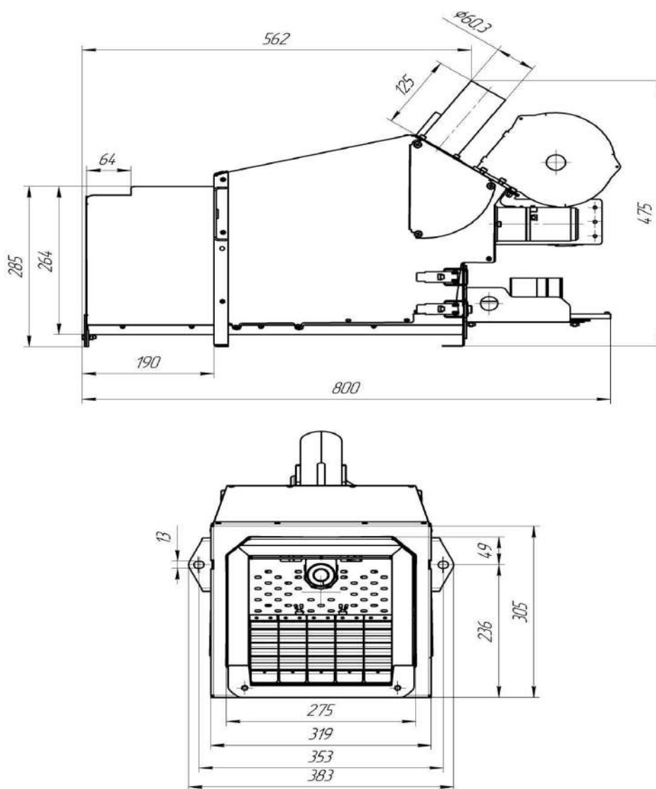
Рис. 1. Габаритные и присоединительные размеры горелки.
