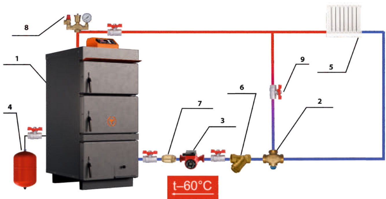
Рисунок 3 – Типовая схема обвязки котла «ТЕПЛОВЪ» с баком аккумулятором
