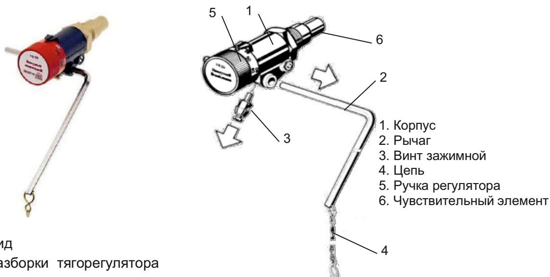
Рисунок 8. Общий вид тягорегулятора
