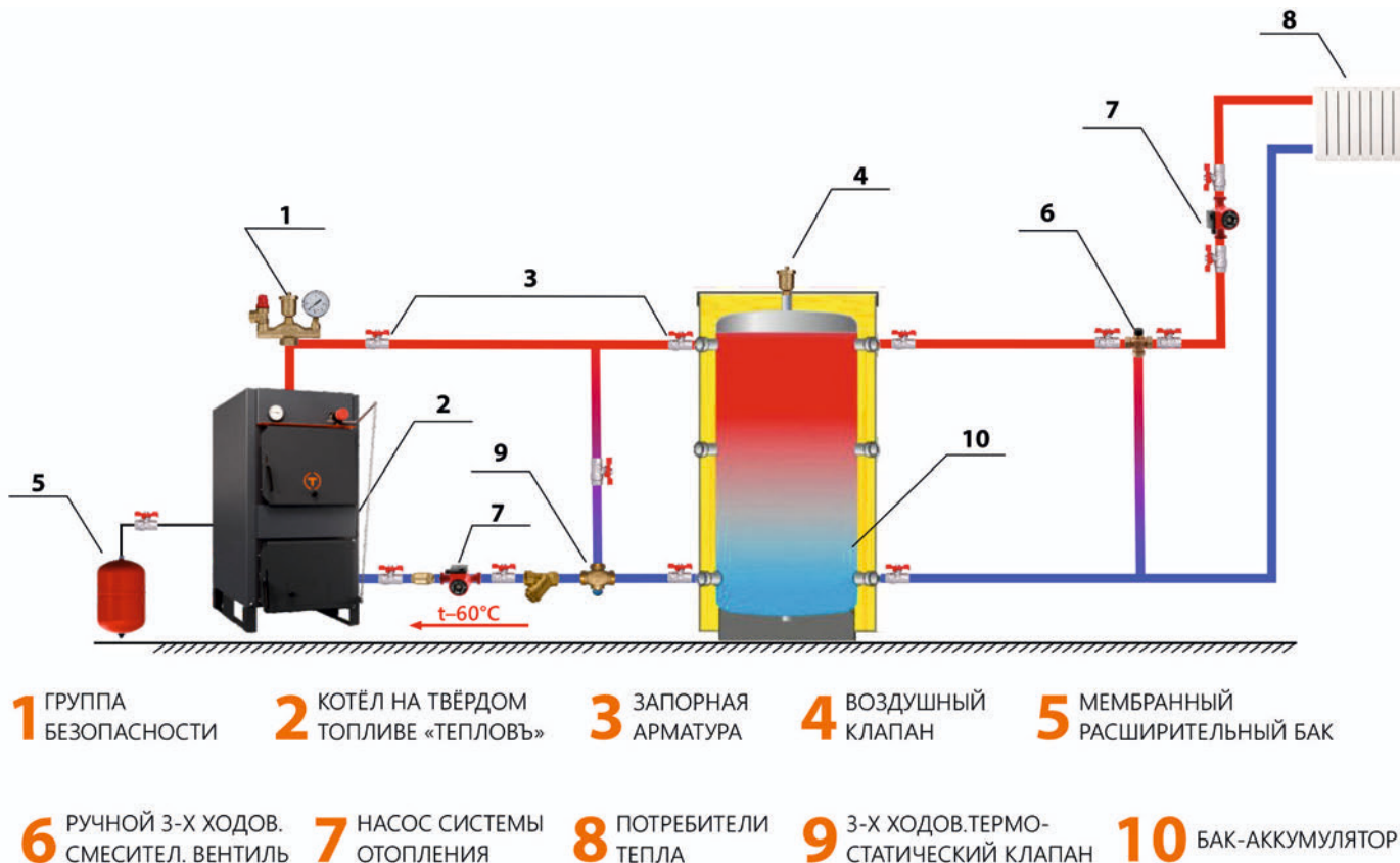
Рисунок 4. Типовая схема обвязки котла «ТЕПЛОВЪ» с бак- аккумулятором
