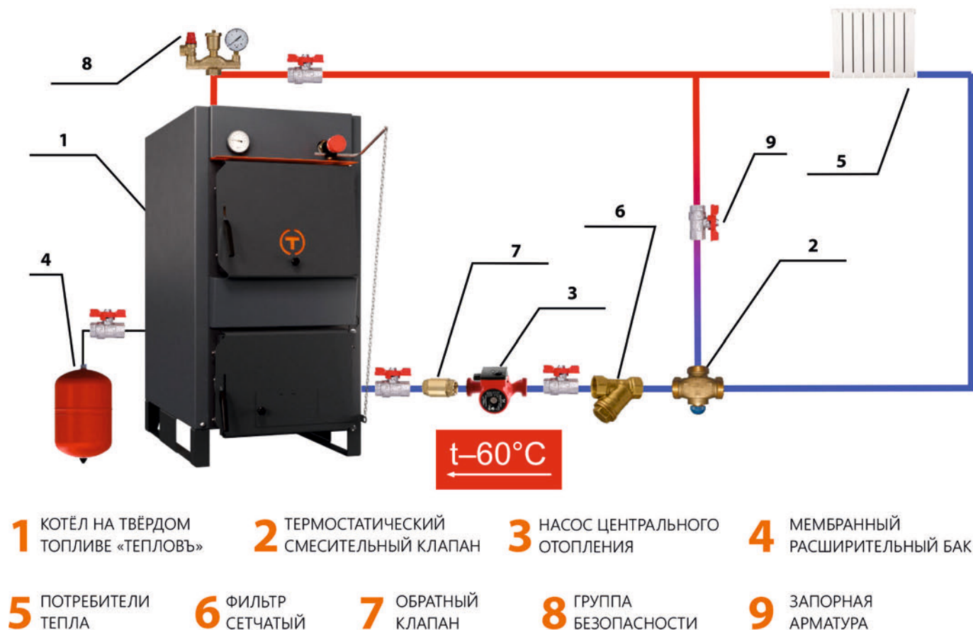
Рисунок 5. Типовая схема обвязки котла «ТЕПЛОВЪ» с 3-х ходовым клапаном
