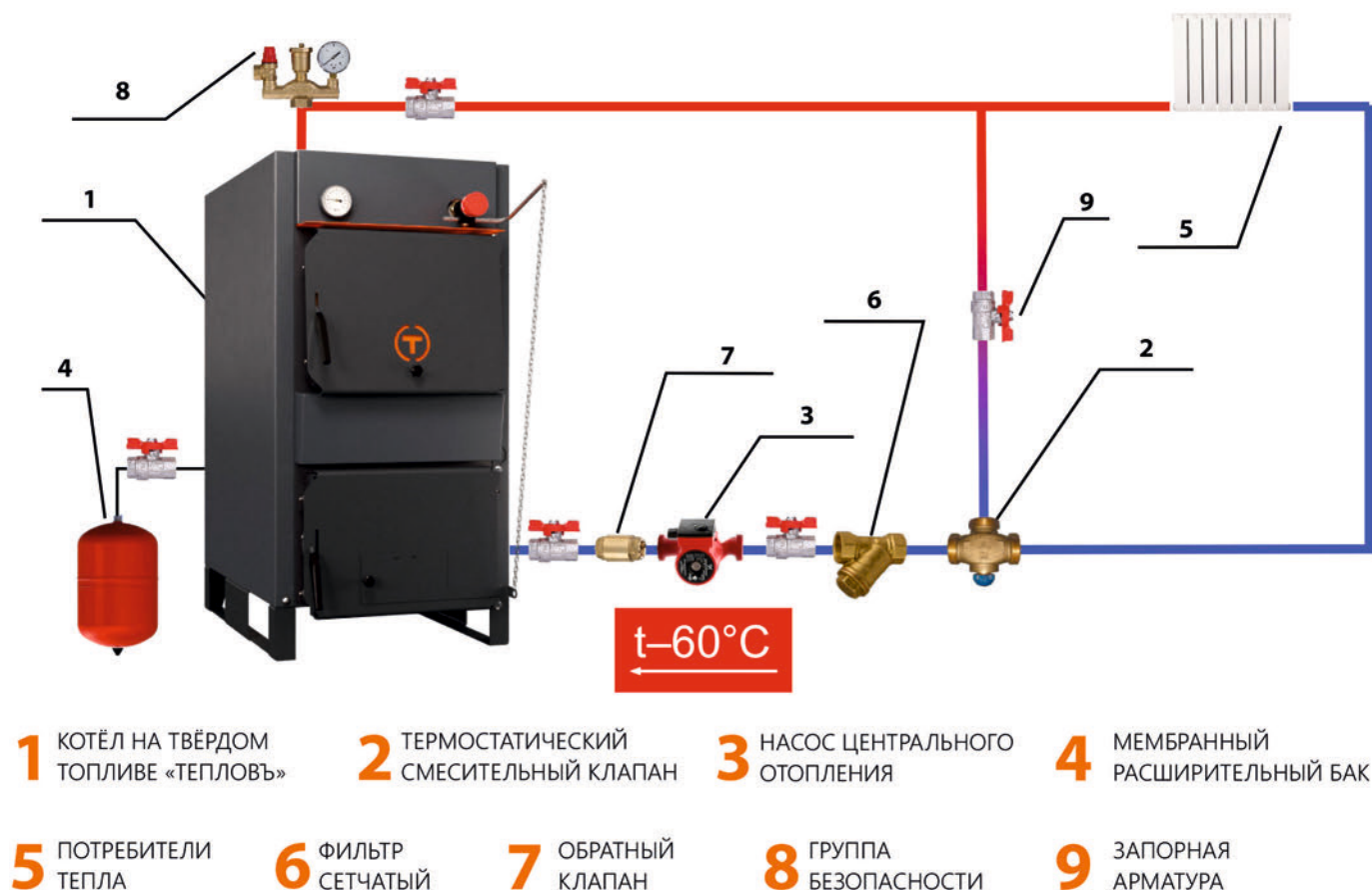
Рисунок 4. Типовая схема обвязки котла «ТЕПЛОВЪ» с 3-х ходовым клапаном
