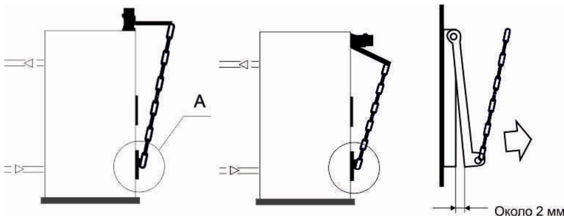
Рисунок 7 – Схема закрепления тягорегулятора на заслонке нижней дверцы Котла
