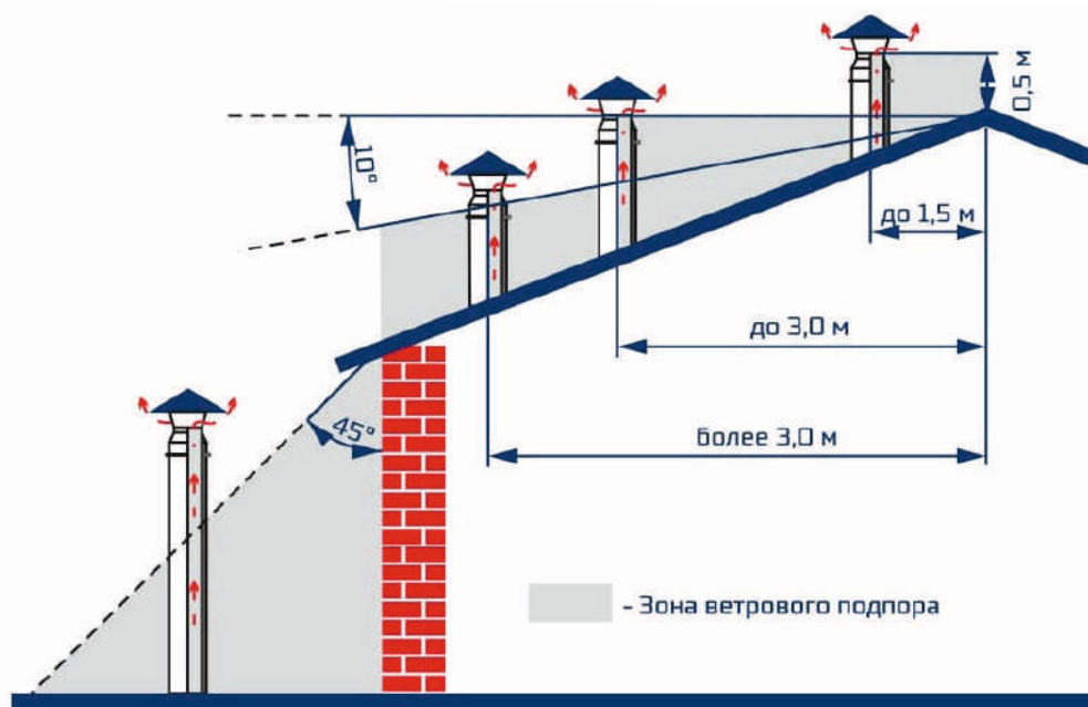
Вылет трубы дымовой трубы в зависимости от конструкции кровли
