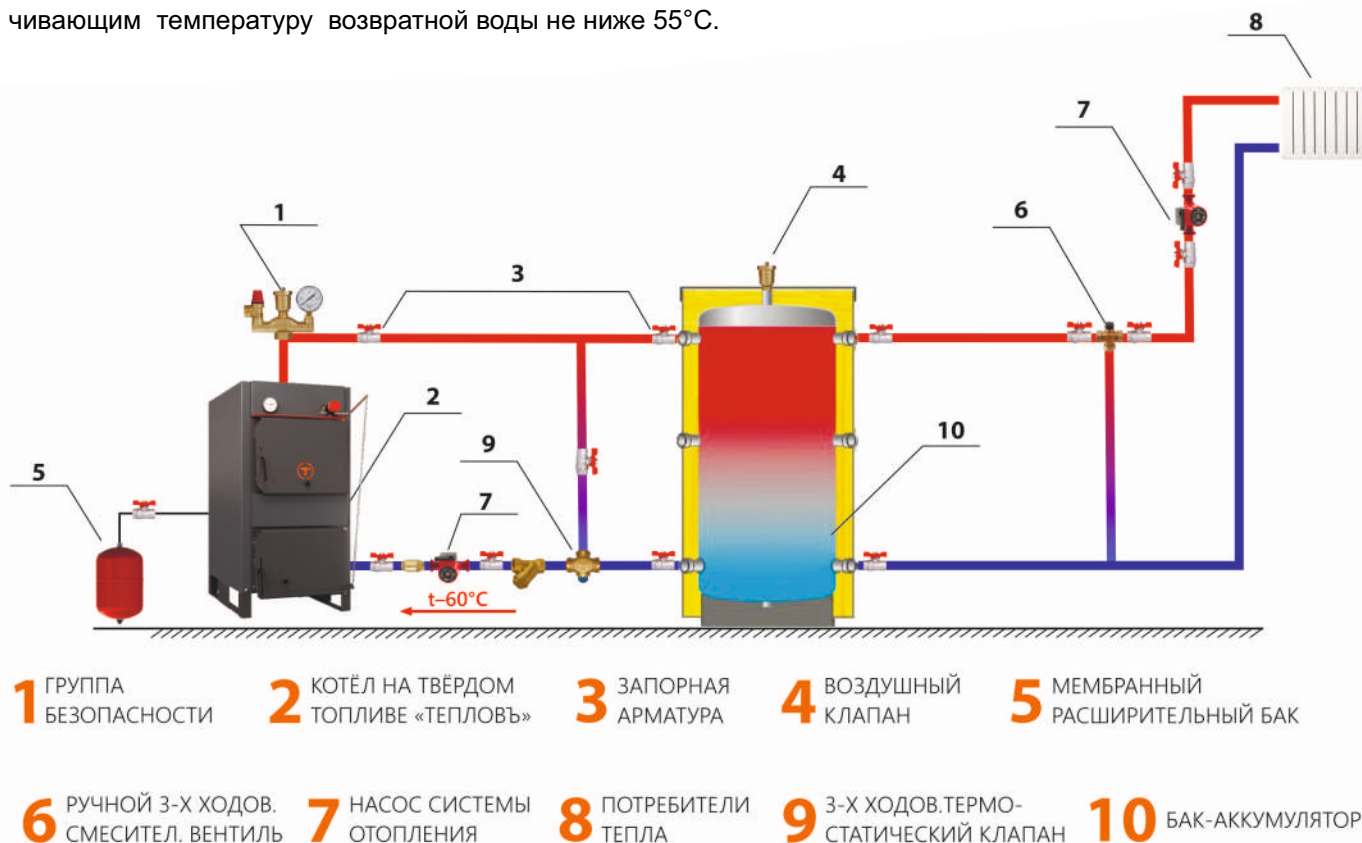
Рисунок 4. Типовая схема обвязки котла с баком-аккумулятором
