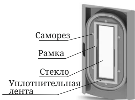
Рисунок 17. Дверца печи Огонь-батарея
