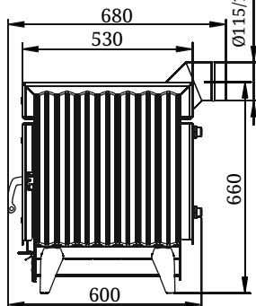
Рисунок 4. Габаритные размеры «Огонь-батарея 7Б» с выходом для трубы назад
