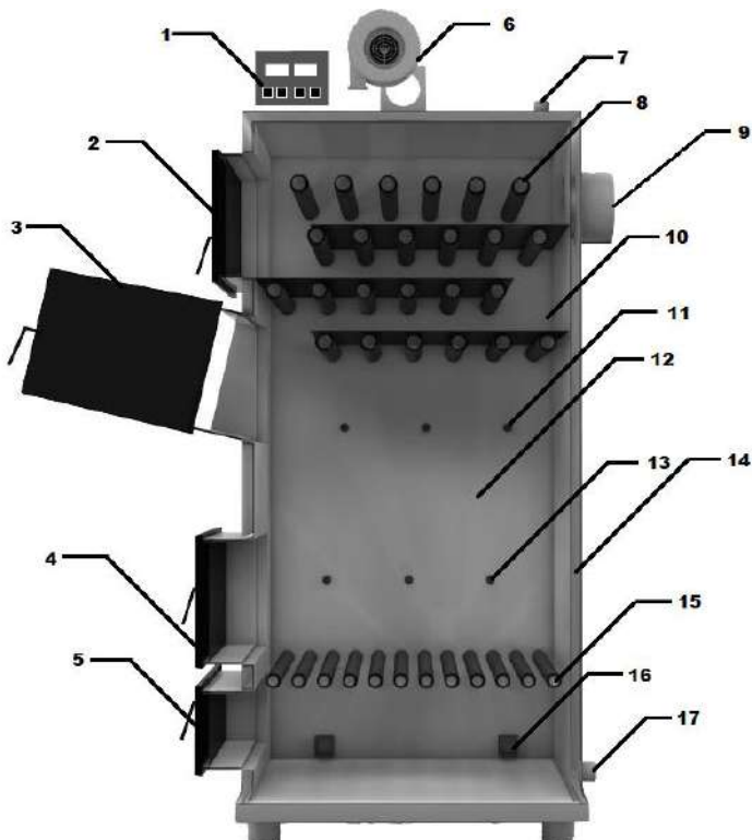
Рис. 1 Строение котла.
