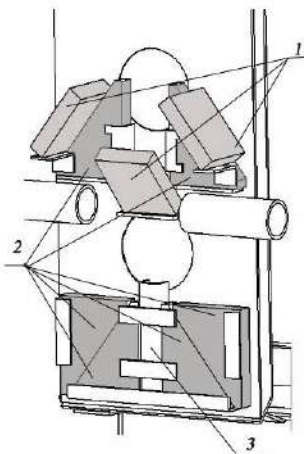
Рис. 11 Укладка шамотных кирпичей для типов 12 и 16
