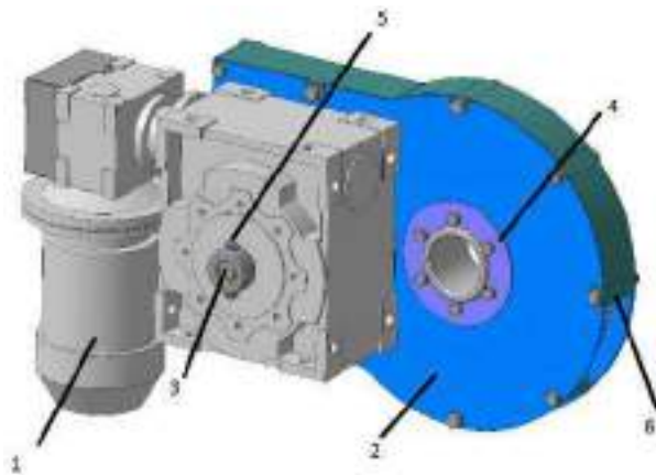
Рис.11 Привод колосника для котлов мощностью 400 – 1500 кВт
