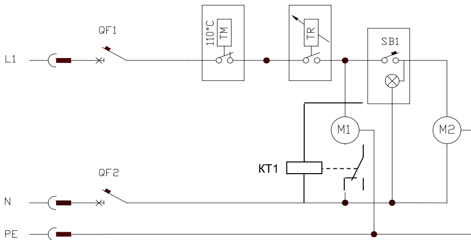
Рис.2 а Схема электрическая принципиальная без ПЧВ
