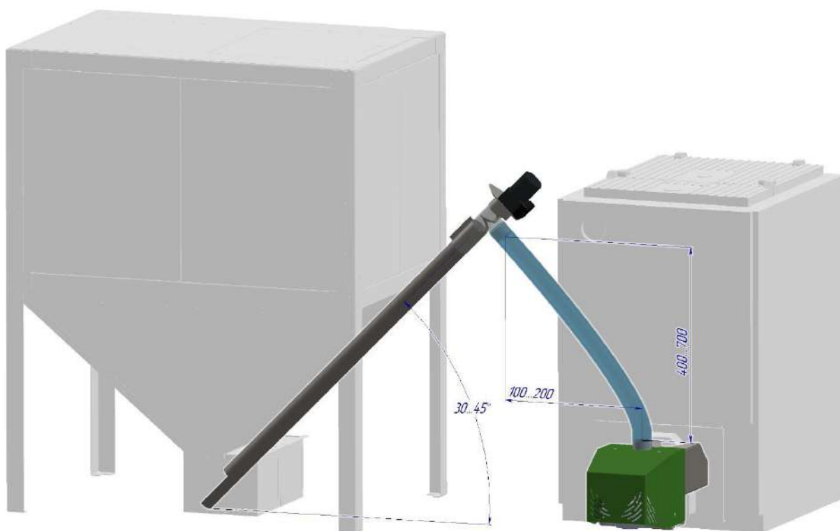
Рис. 3 – Пример установки шнекового питателя
