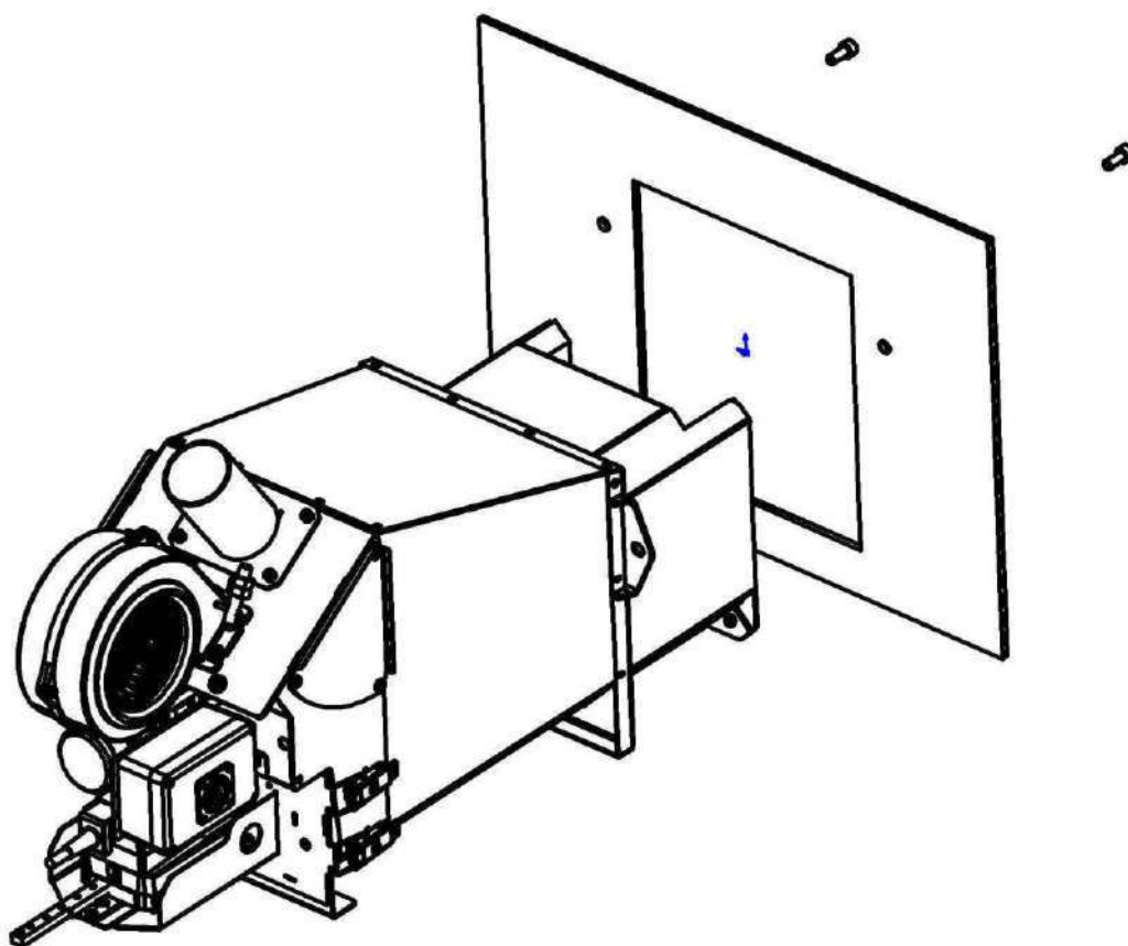
Рис. 6 – Установка горелки
