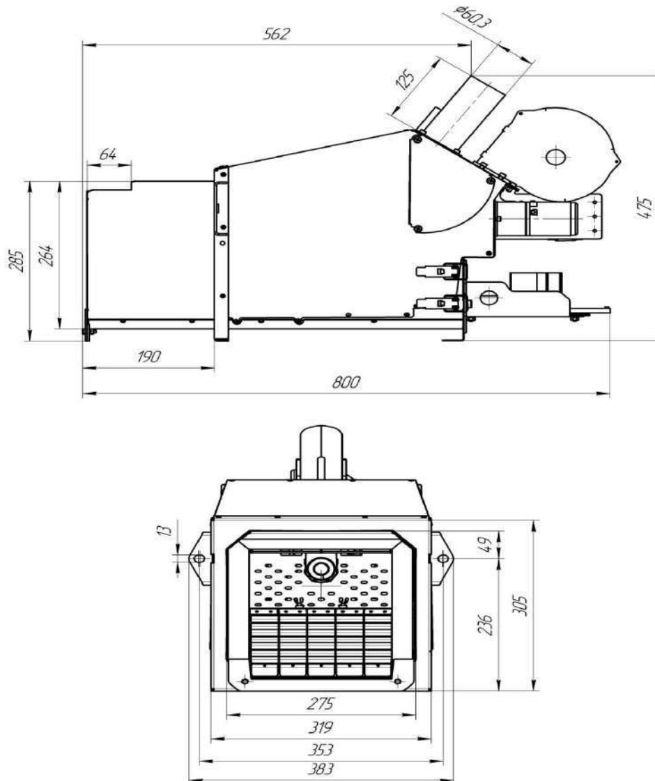
Рис. 1. Габаритные и присоединительные размеры горелки.
