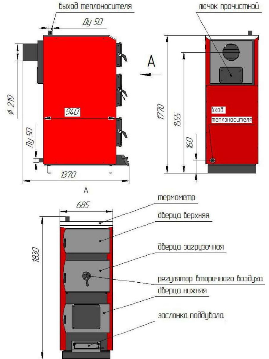
Рисунок 3. Основные размеры и элементы котлов DRAGON-KR
