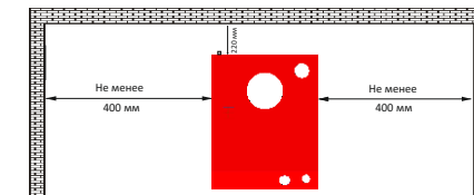
Рисунок 4. Установка котла в помещении котельной.
