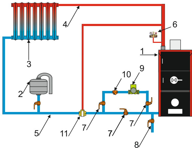
1-котел
