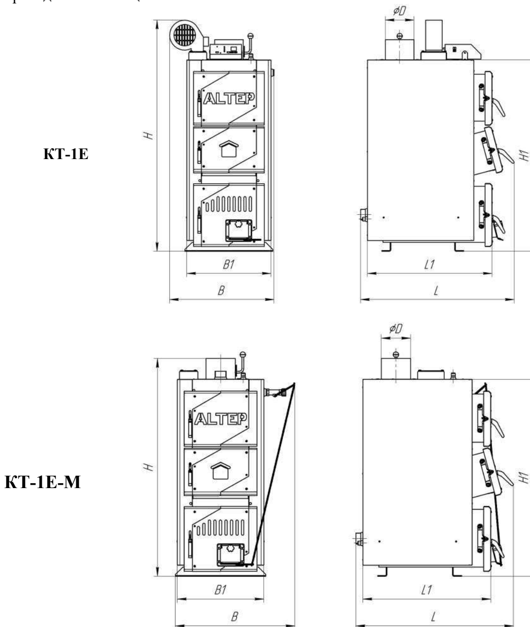
Рисунок 1 – Габаритный чертёж котла типа КТ-1Е (М)
