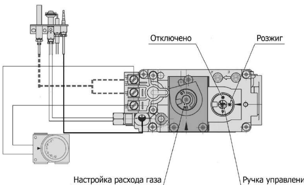
Рисунок 3 – Элементы управления на газовом блоке 820 NOVA mV
