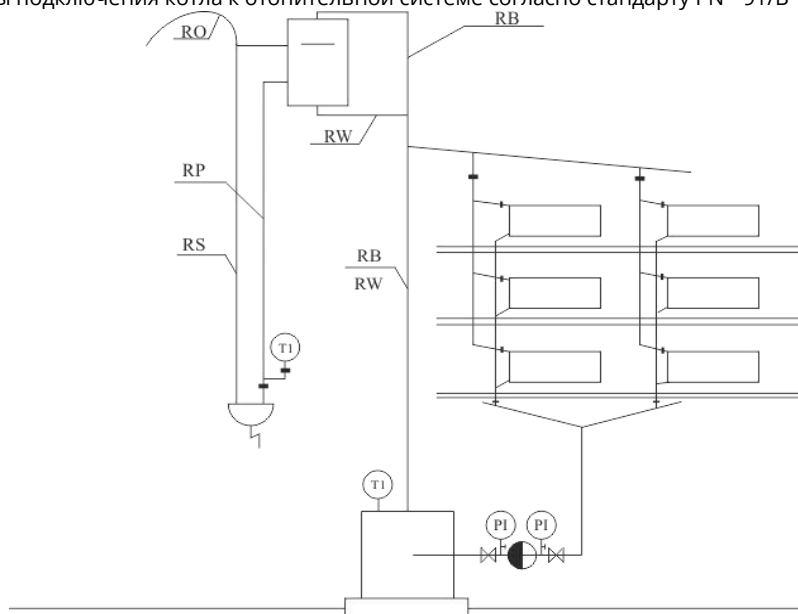
Рисунок 14.1 Схема подключения котла к системе отопления
