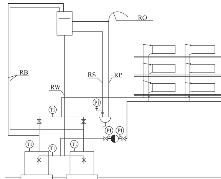
Рисунок 14.2 Схема подключения котла к системе отопления
