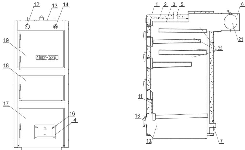
Рисунок 8.3 Основные конструктивные элементы котлов SE 120 – 250
