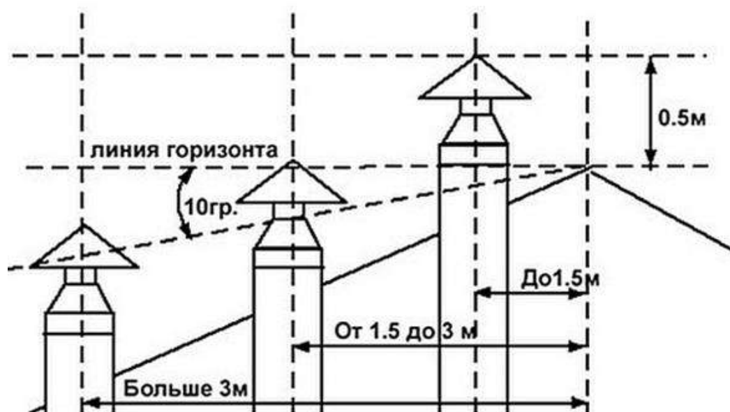
Рисунок 12 — Схема размещения дымоходов.
