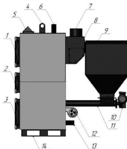
Рисунок 8 – Схема размещения составных элементов в котлах серии F-VARM GE Z (вид сбоку). 1-дверца теплообменника; 2-дверца горелки; 3-дверца зольника; 4-ухо транспортировочное; 5-контроллер; 6-труба подачи; 7-дымовая труба; 8-короб дымохода; 9-бункер; 10-мотор-редуктор; 11-труба топливоподачи; 12-вентилятор наддува; 13-труба обратной линии; 14-опора котла.
