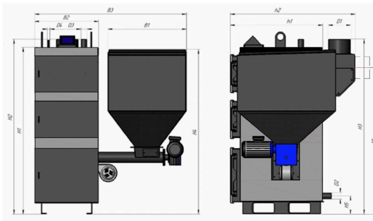
Рисунок 1. Габаритные размеры F-VARM GE.
