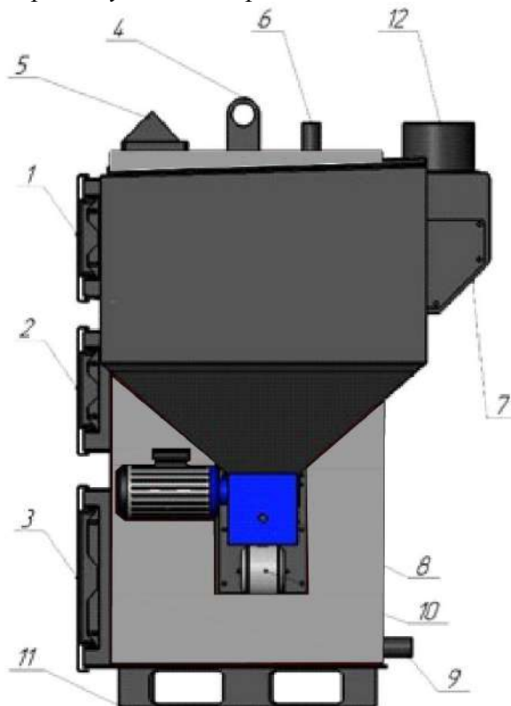
Рисунок 5. Схема размещения составных элементов в котлах серии F-VARM GE (вид с фронта). 1-дверца теплообменника; 2-дверца горелки; 3-дверца зольника; 4-ухо транспортировочное; 5-контроллер; 6-труба подачи; 7-бункер; 8-мотор-редуктор; 9-труба топливоподачи; 10-вентилятор наддува; 11-опора котла.
