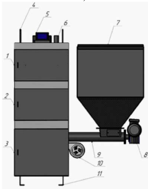
Рисунок 5. Схема размещения составных элементов в котлах серии F-VARM GE (вид с фронта). 1-дверца теплообменника; 2-дверца горелки; 3-дверца зольника; 4-ухо транспортировочное; 5-контроллер; 6-труба подачи; 7-бункер; 8-мотор-редуктор; 9-труба топливоподачи; 10-вентилятор наддува; 11-опора котла.
