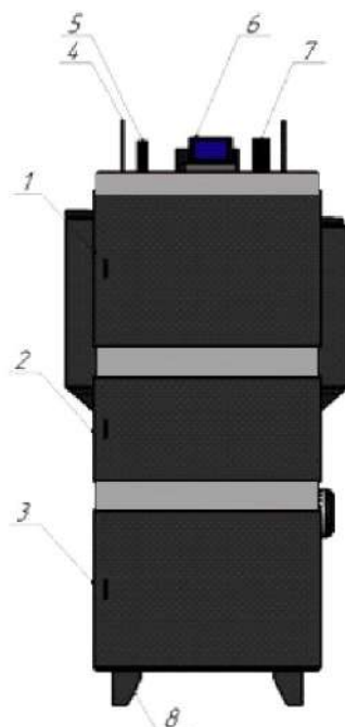
Рисунок 7 — Схема размещения составных элементов в котлах серии F-VARM GE Z вид с фронта). 1-дверца теплообменника; 2-дверца горелки; 3-дверца зольника; 4-ухо транспортировочное; 5-группа безопасности; 6-контроллер; 7-труба подачи; 8-опора котла
