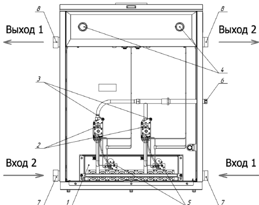
Рис. 1.2. Котёл «Премиум ПРО» 90; 100 с автоматикой 820 Nova
