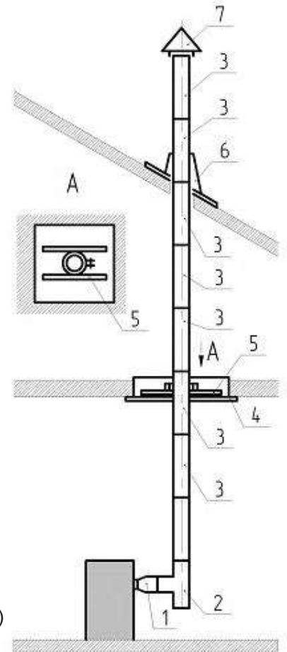
Рисунок Б.1. Пример сборки утепленного (сэндвич) дымохода по конденсату внутри и снаружи помещения
