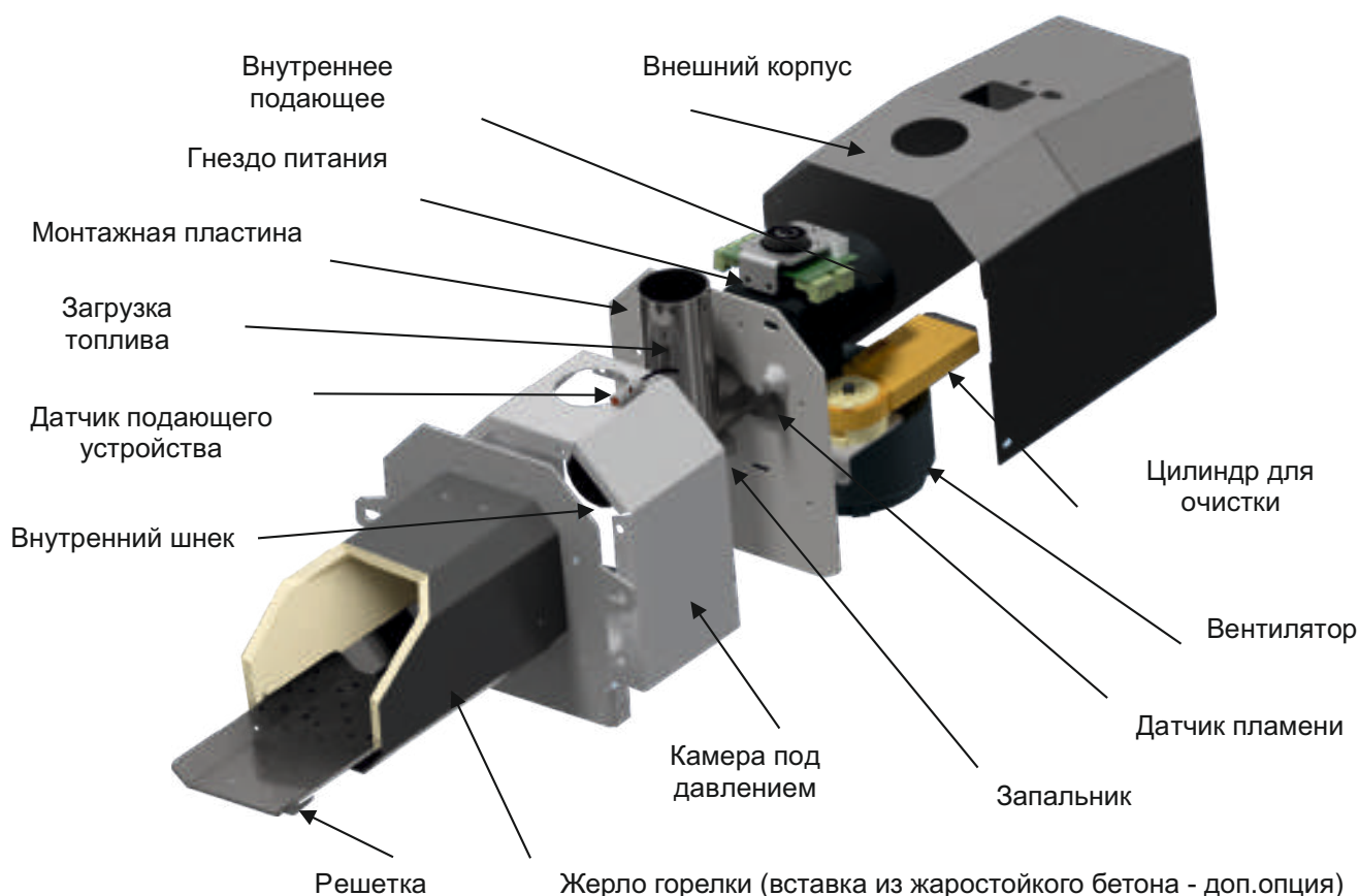
Рисунок 6. Состав Горелок Lавого Eco 25-100
