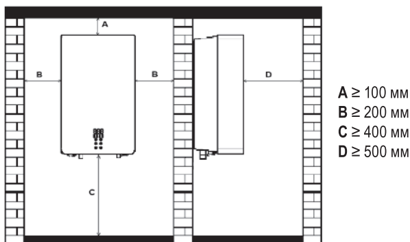
Рисунок 4 - Минимальные свободные расстояния от поверхностей до корпуса котла
