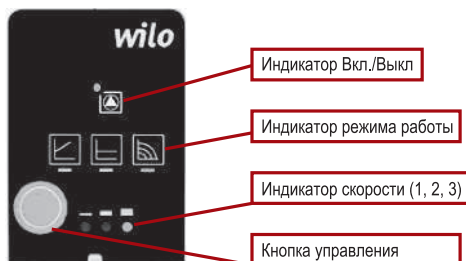
Рисунок 7 - Панель управления насосом Wilo PARA
