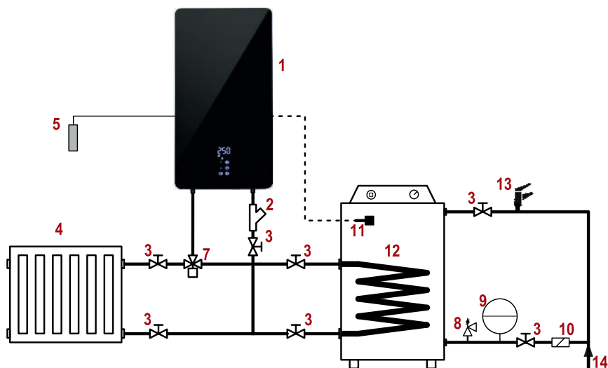
Рисунок 22 - Схема подключения к котлу бойлера ГВС
