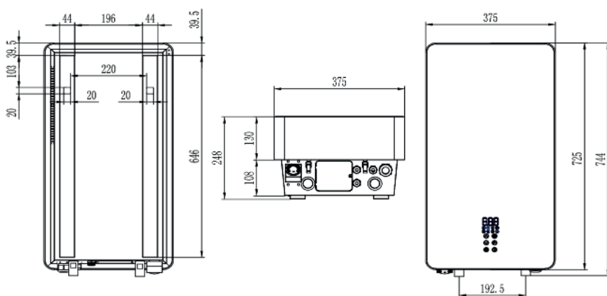
Рисунок 6 - Основные размеры
