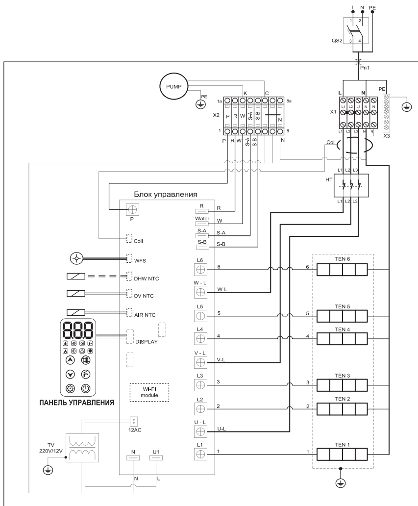
Рисунок 14 - Схема подключения котлов PROPLUS 4,5 кВт, 6 кВт и 7,5 кВт к однофазной сети 220В (50Гц)
