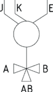
Рисунок 24 - Электроподключение привода трехходового клапана
