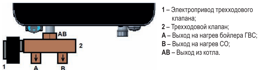
Рисунок 23 - Установка трехходового клапана на патрубке выхода из котла
