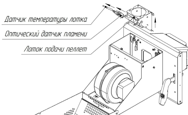
Рисунок 13 Замена лотка загрузочного
