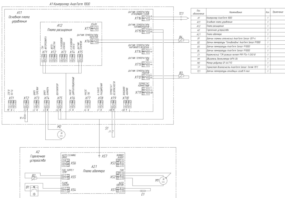
Рисунок 5 Схема электрических соединений контроллера
