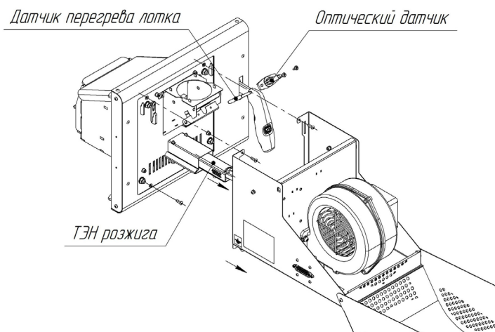
Рисунок 16 Демонтаж кожуха горелки, датчиков и ТЭНа
