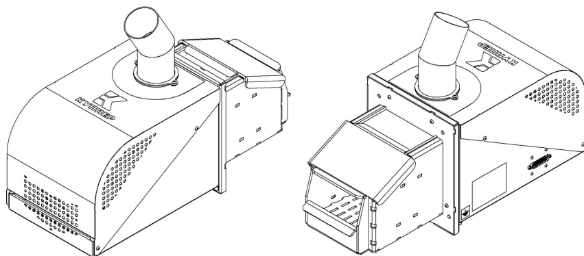
Рисунок 21 Горелочное устройство (без двери)
