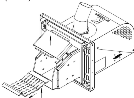
Рисунок 12 Чистка горелочного устройства
