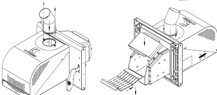
Рисунок 4. Установка загрузочного патрубка, колосника и крышки жаровни
