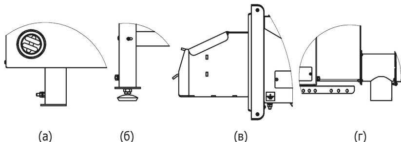
Рисунок 8 Размещение болта заземления
