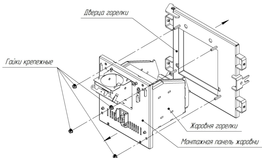
Рисунок 18 Демонтаж двери
