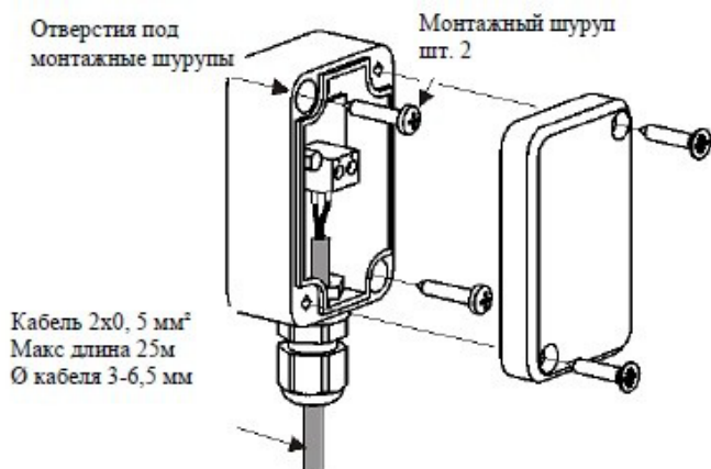
Рисунок 7 Погодный датчик
