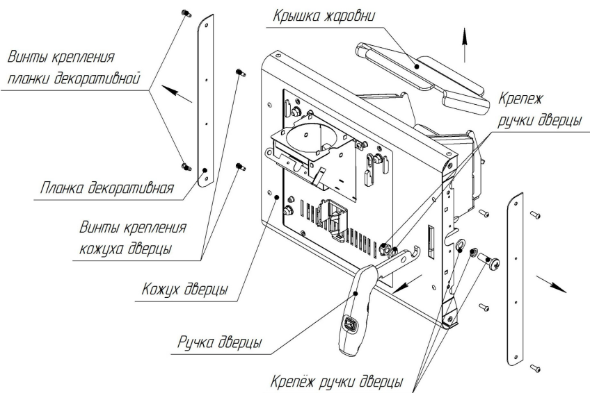
Рисунок 17 Демонтаж кожуха двери, ручки и крышки жаровни
