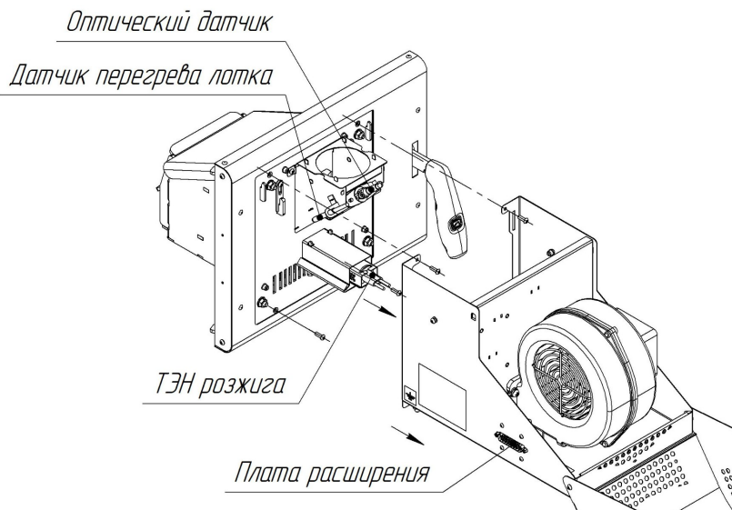
Рисунок 15 Замена ТЭНа розжига
