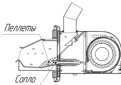
Рисунок 11 Ручная загрузка топлива для розжига
