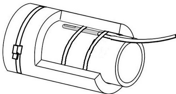
Рисунок 6 Установка датчика температуры и теплоизолирующей гильзы
