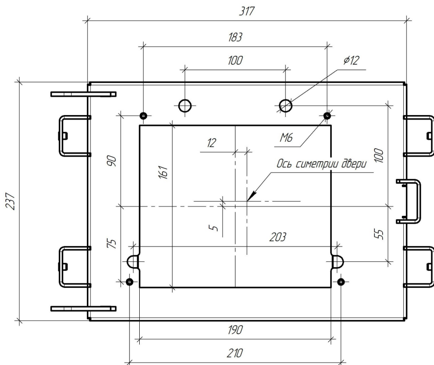
Рисунок 20 Разметка проема и мест крепления ГПФ-42 (3.0)
