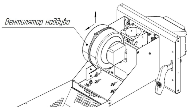
Рисунок 14 Замена вентилятора наддува
