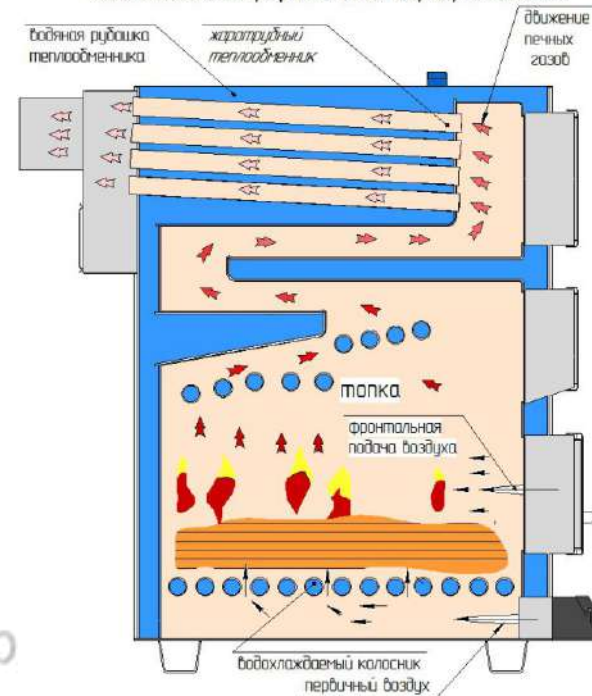
Схема теплообмена при работе котла на резервном топливе
