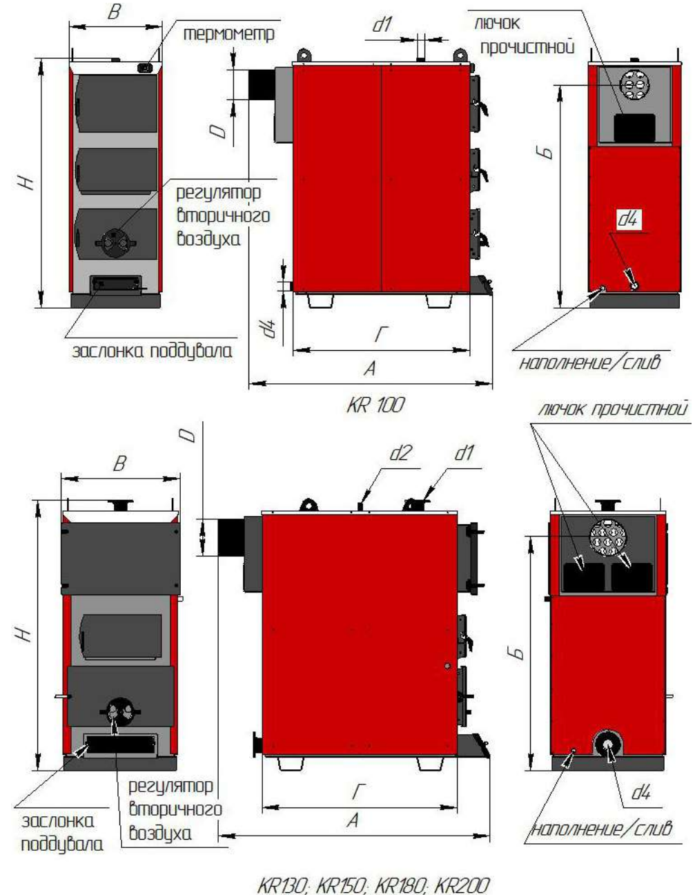
Рисунок 3. Основные размеры котлов HOT DRAGON-KR
