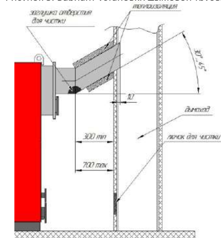
Рисунки 5. Варианты установки дымовой трубы
