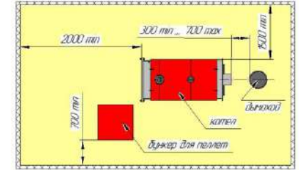
Рисунок 4. Установка котла в помещении котельной.
