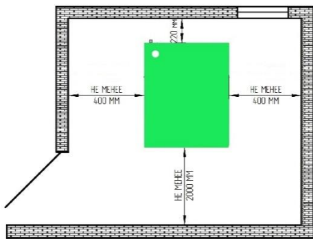
Рис. 4. Установка котла в помещении котельной
