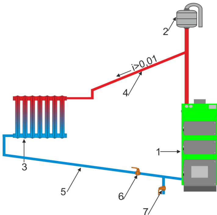
Рис. 2.1. Вариант схемы присоединения котла к системе отопления открытого типа
