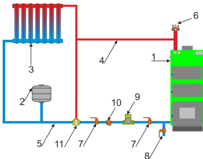
Рис. 2.2. Вариант схемы присоединения котла к системе отопления закрытого типа
