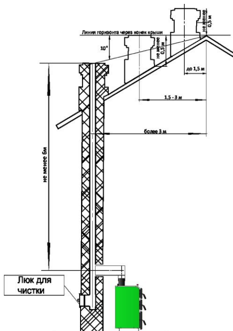
Рисунок 5. Варианты установки дымовой трубы
