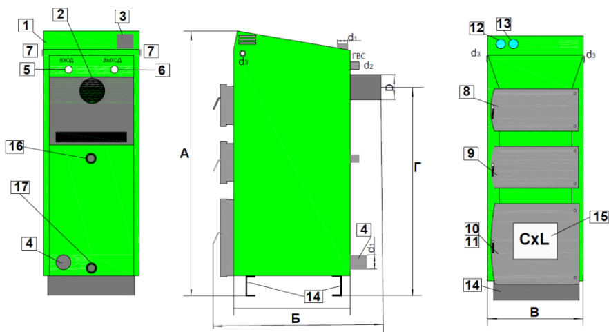
Рисунок 3. Основные размеры и элементы котлов Hot Dragon BIO(SBE/SBLE)
