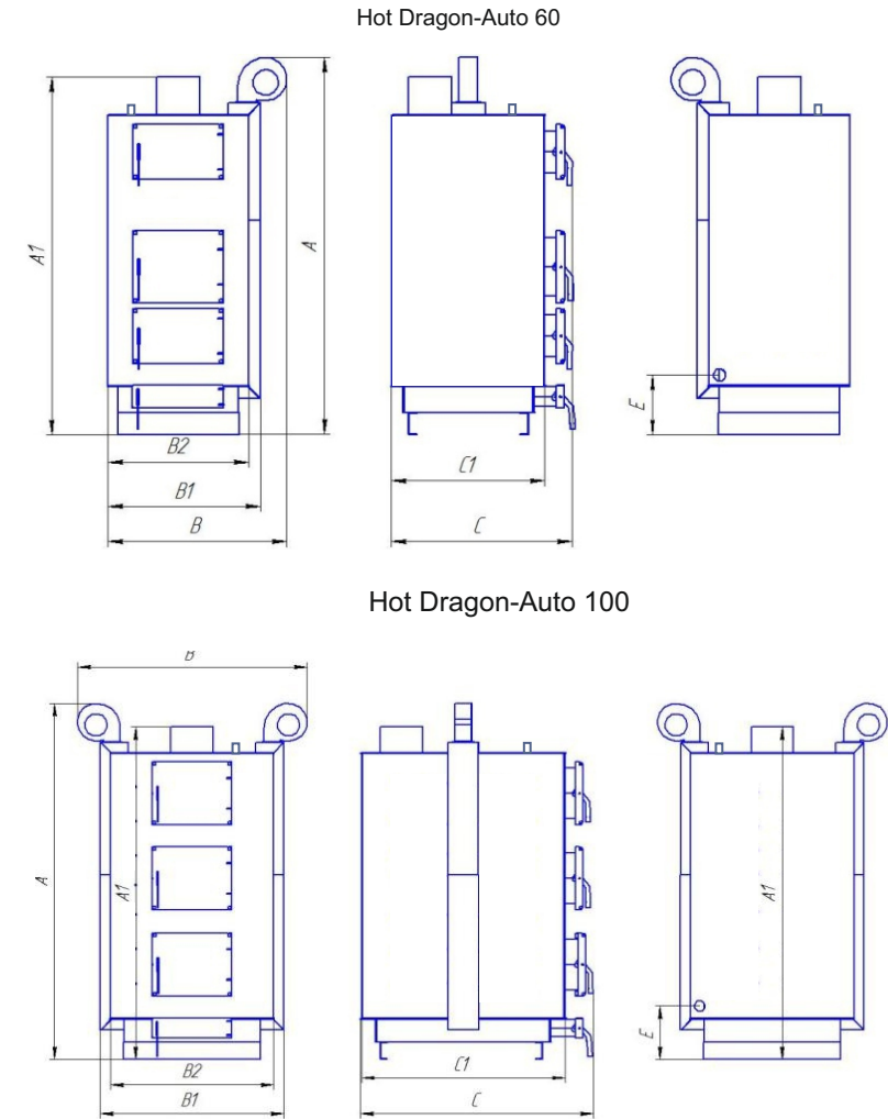
Рисунок 3. Основные размеры котлов HOT DRAGON-Auto
