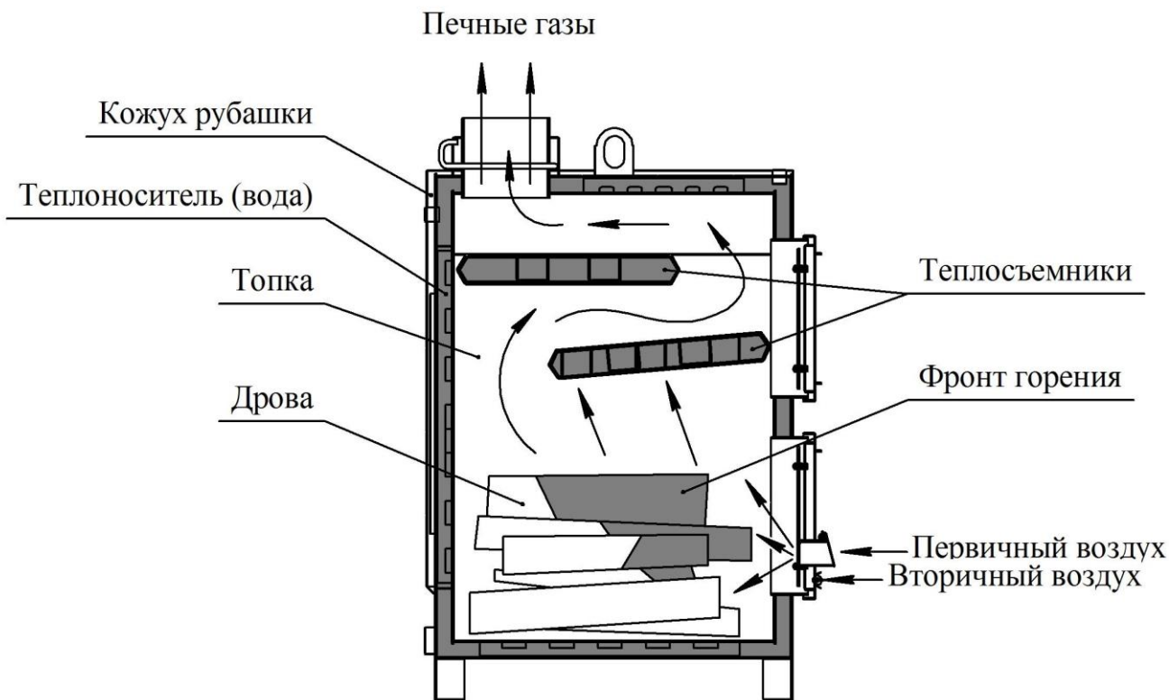
Рисунок 1 – Схема КОД-50
