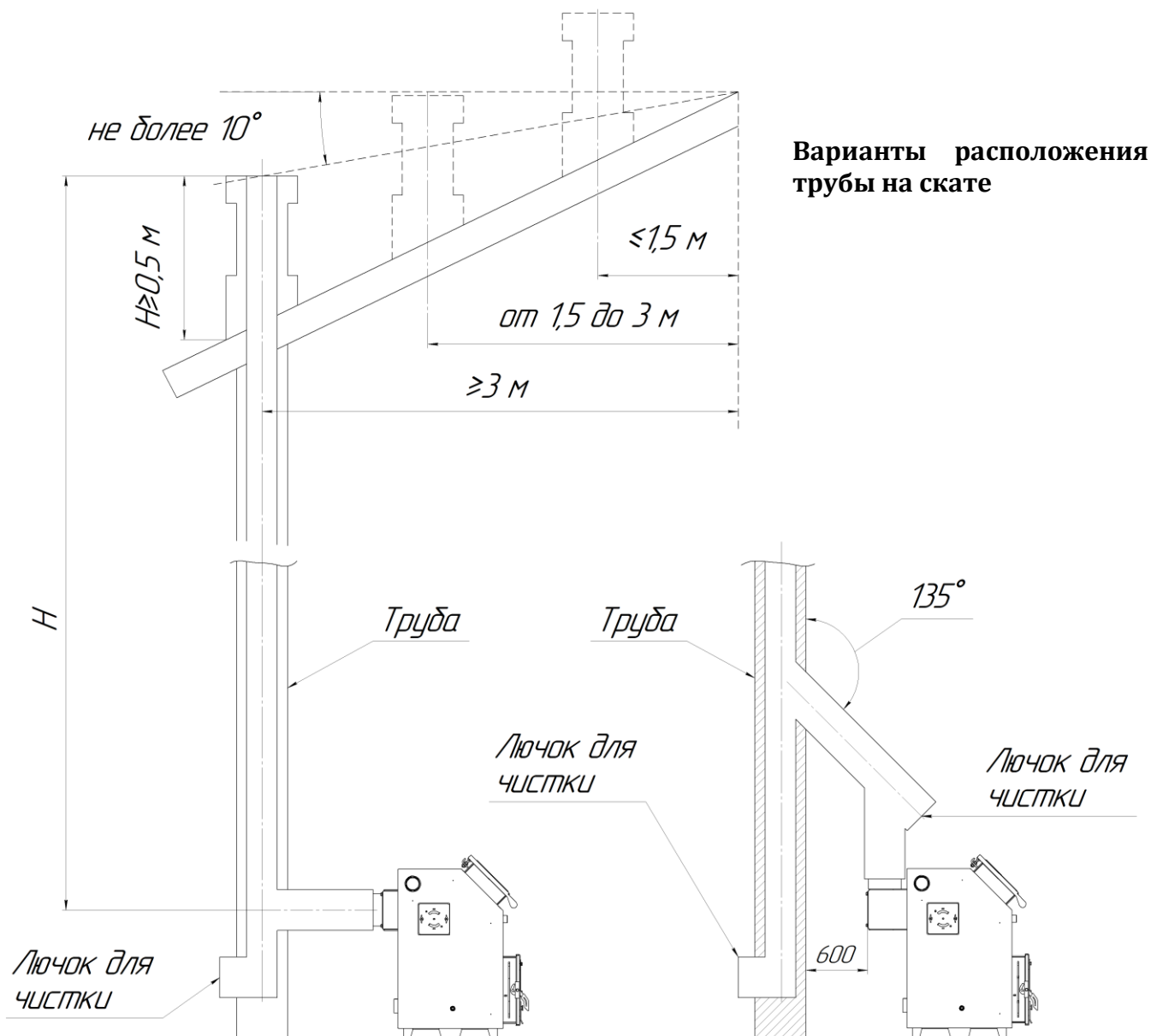
Рисунок 5 – Подключение котла к дымовой трубе (2 варианта)
