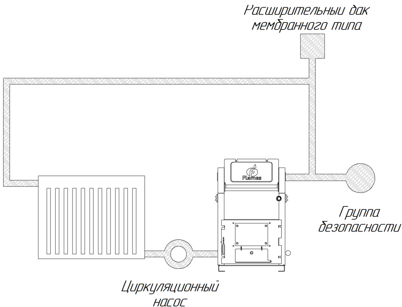
Рисунок 9 – Схема закрытой системы отопления с принудительной циркуляцией
