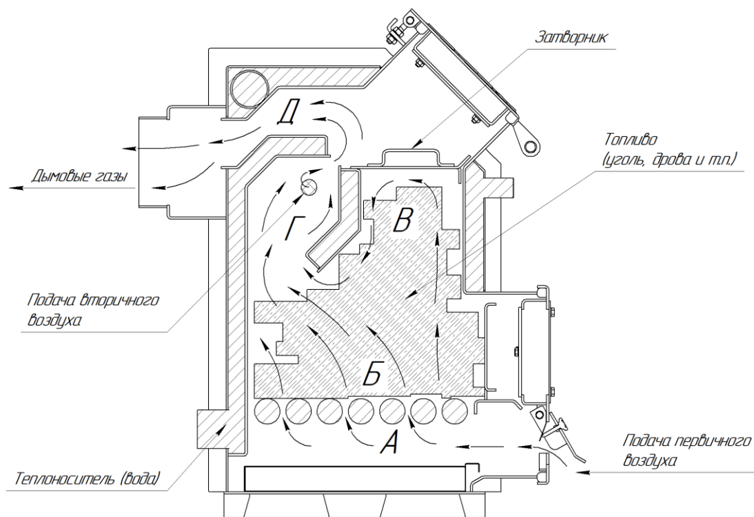
Рисунок 1 – Схема движения газов в котле
