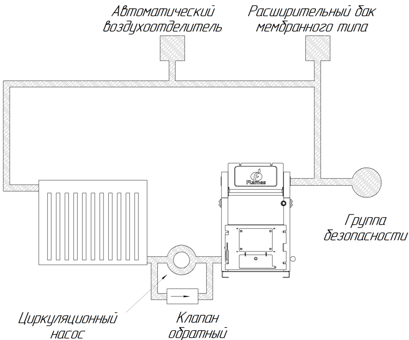
Рисунок 10 – Схема закрытой системы со смешенной циркуляцией
