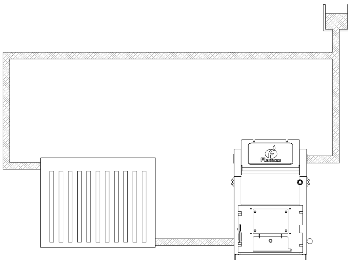
Рисунок 8 – Схема открытой системы отопления с естественной циркуляцией
