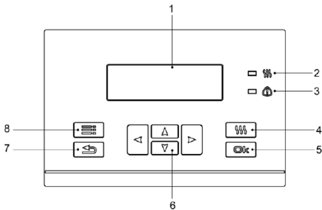
Рисунок 2. Блок управления
