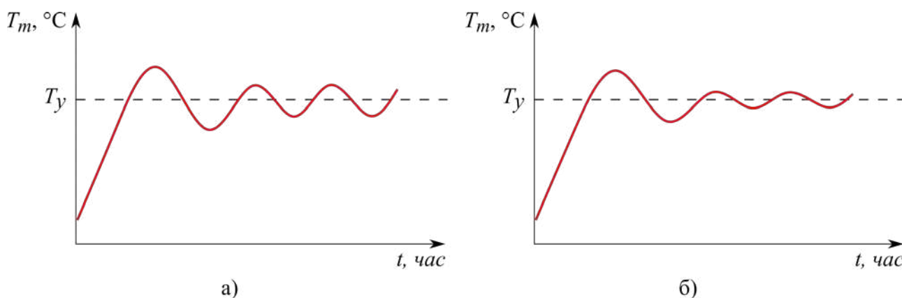
Рисунок 3: Колебания температуры котла в зависимости от значений коэффициентов AirFlow ( T_t — температура теплоносителя, T_y — температура уставки): а) не правильный режим — коэффициент воздуха слишком большой б) правильная настройка
