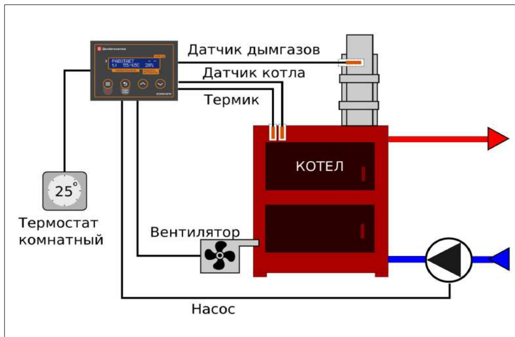
Рисунок 2 - Схема подключения контроллера ECO100 к котлу.
