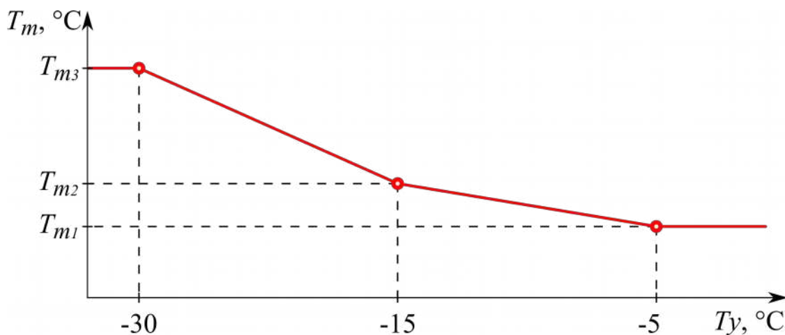
Рисунок 6 - Зависимость температуры теплоносителя от уличной температуры ( T_m — температура теплоносителя (температура котла), T_y — уличная температура)
