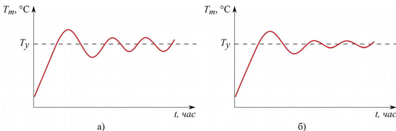
Рисунок 3 - Колебания температуры котла в зависимости от значений коэффициентов вентилятора ( T_m — температура котла, T_y — температура уставки): а) K_V = 70 , K_{VT} = 0 ; б) K_V = 70 , K_{VT} = 30
