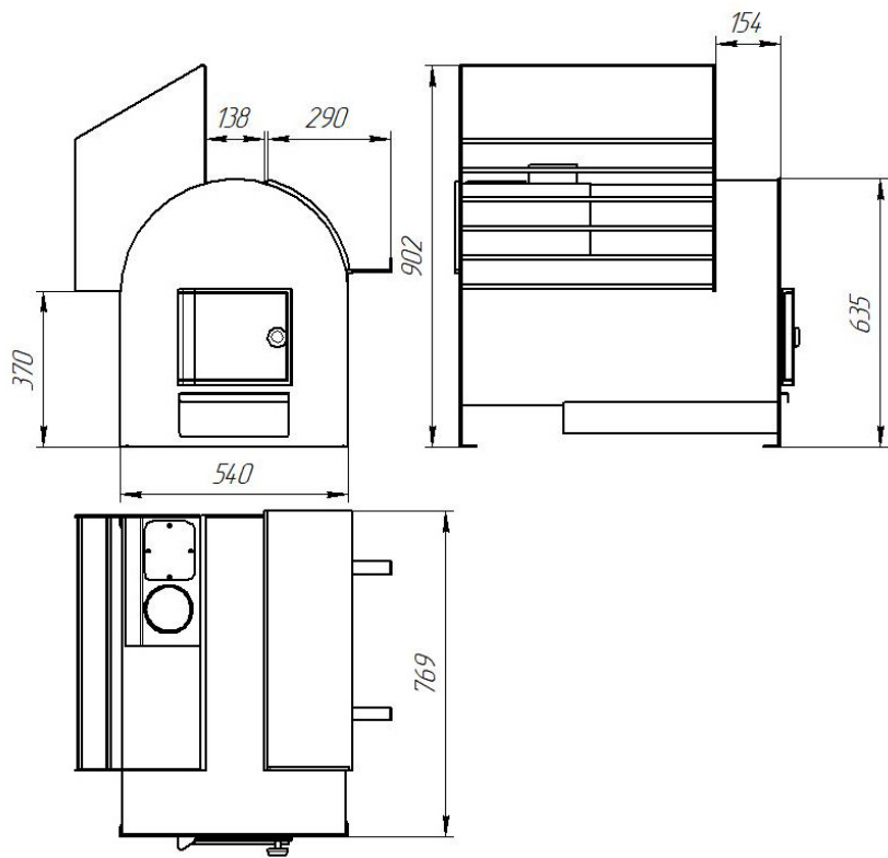
Рисунок 1. Размеры банной печи «Бизон Квадра».
