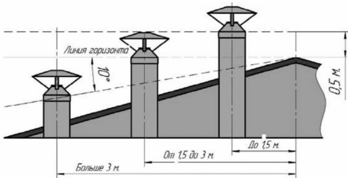
Рисунок 3. Высота дымоходной трубы.
