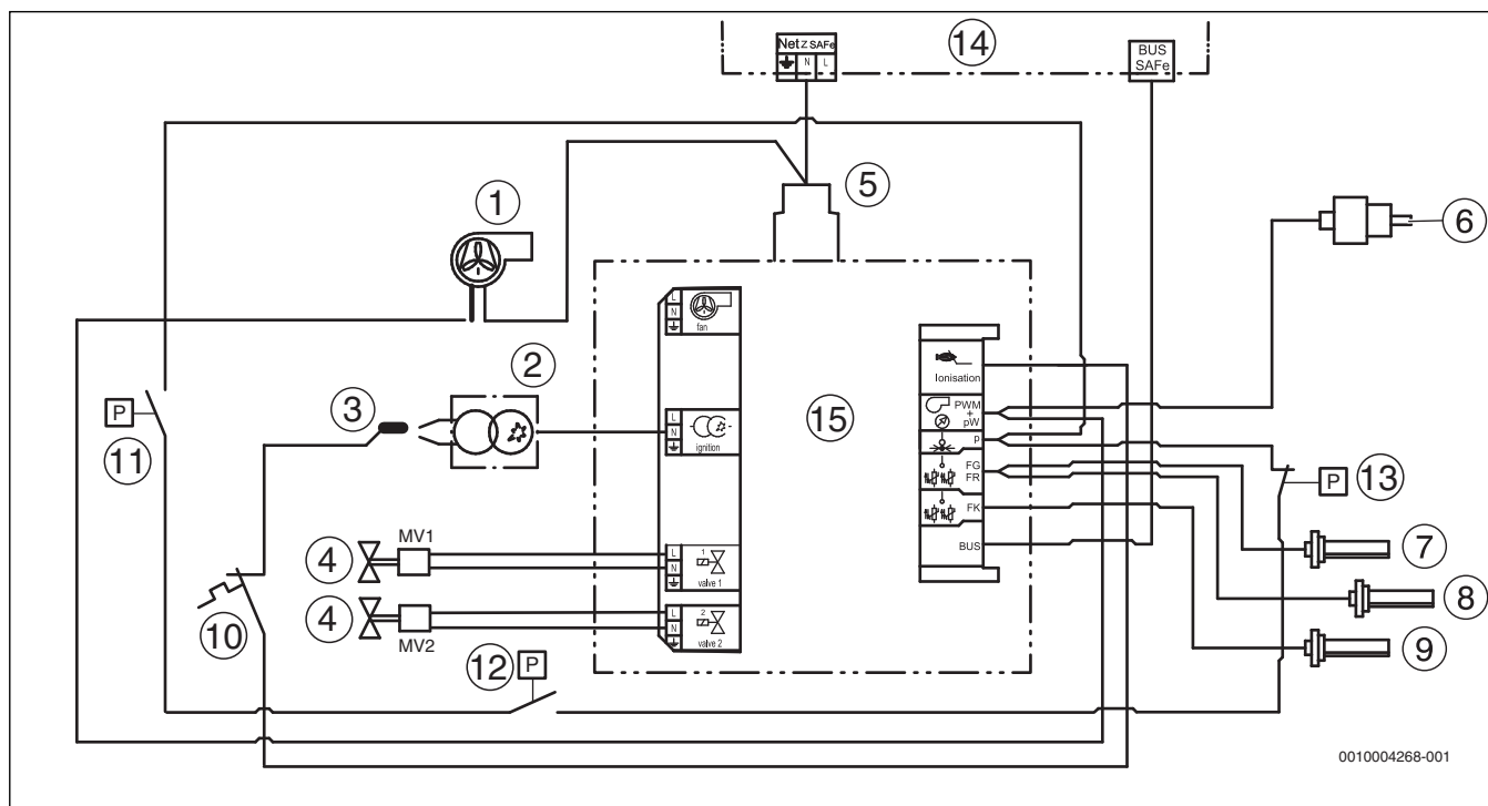
Рис. 72 Схема соединений автомата горения
