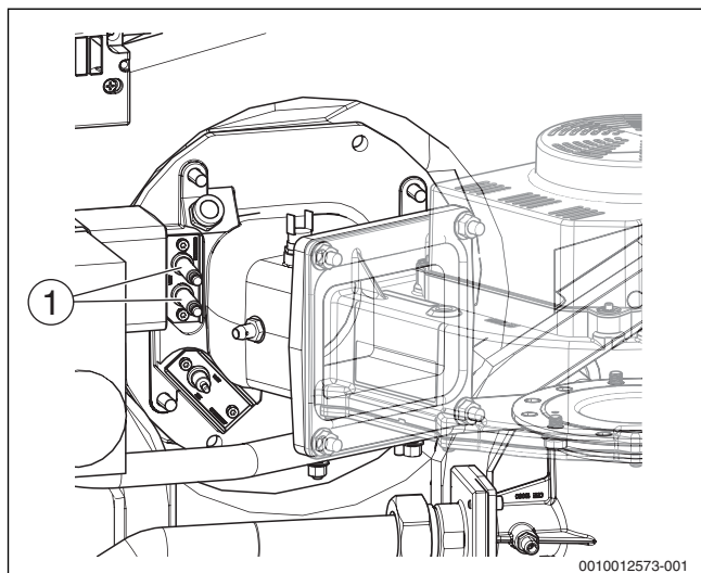
Рис. 38 Запальные электроды
