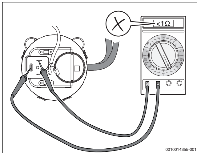
Рис. 70 Измерение электрического сопротивления на контактах дифференциального реле давления (реле неисправно )
