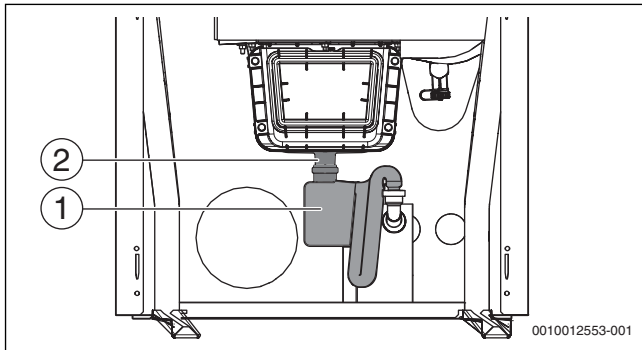
Рис. 46 Демонтаж сифона
