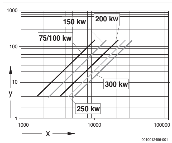
Рис. 71 Гидравлическое сопротивление греющего контура
