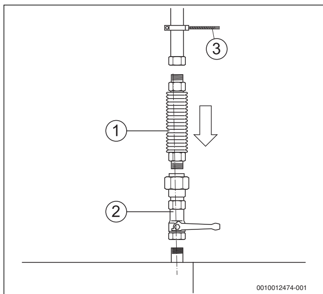
Рис. 22 Подключение газа
