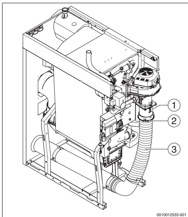
Рис. 41 Канал приточного воздуха
