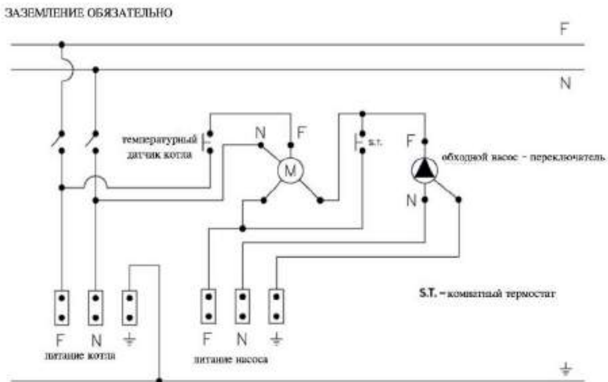
Электрическая схема 2
