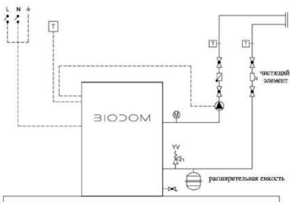
Схема подключения 1
