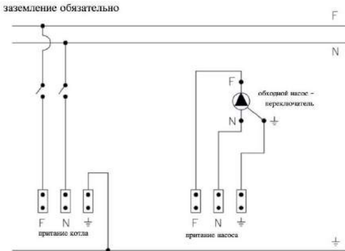
Электрическая схема 3
