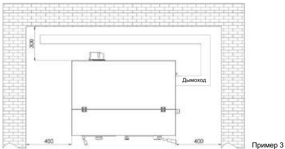
Рис. 1: Минимальное расстояние между котлом и стенами котельной
