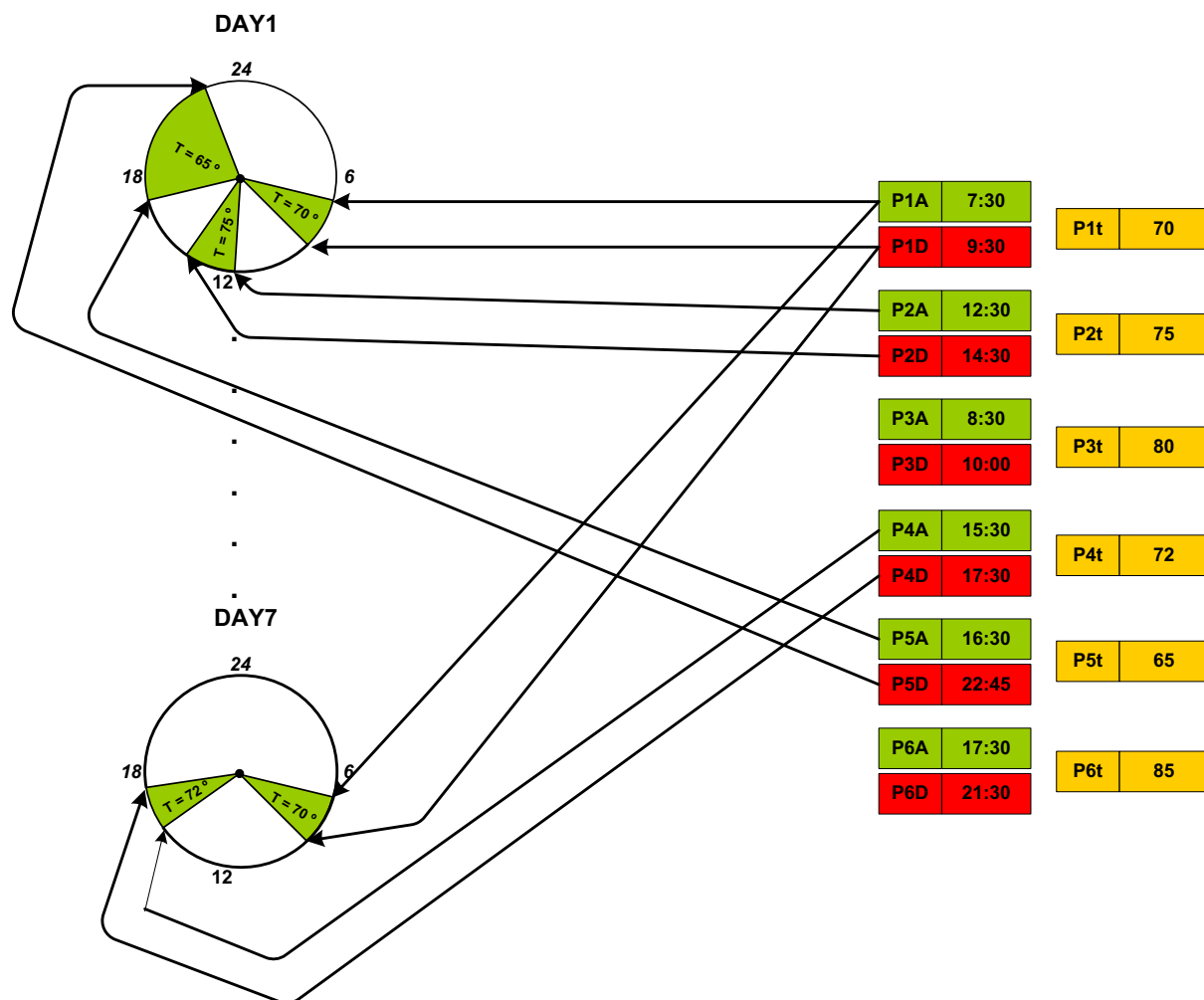
Рисунок 12: Схема настроек таймера
