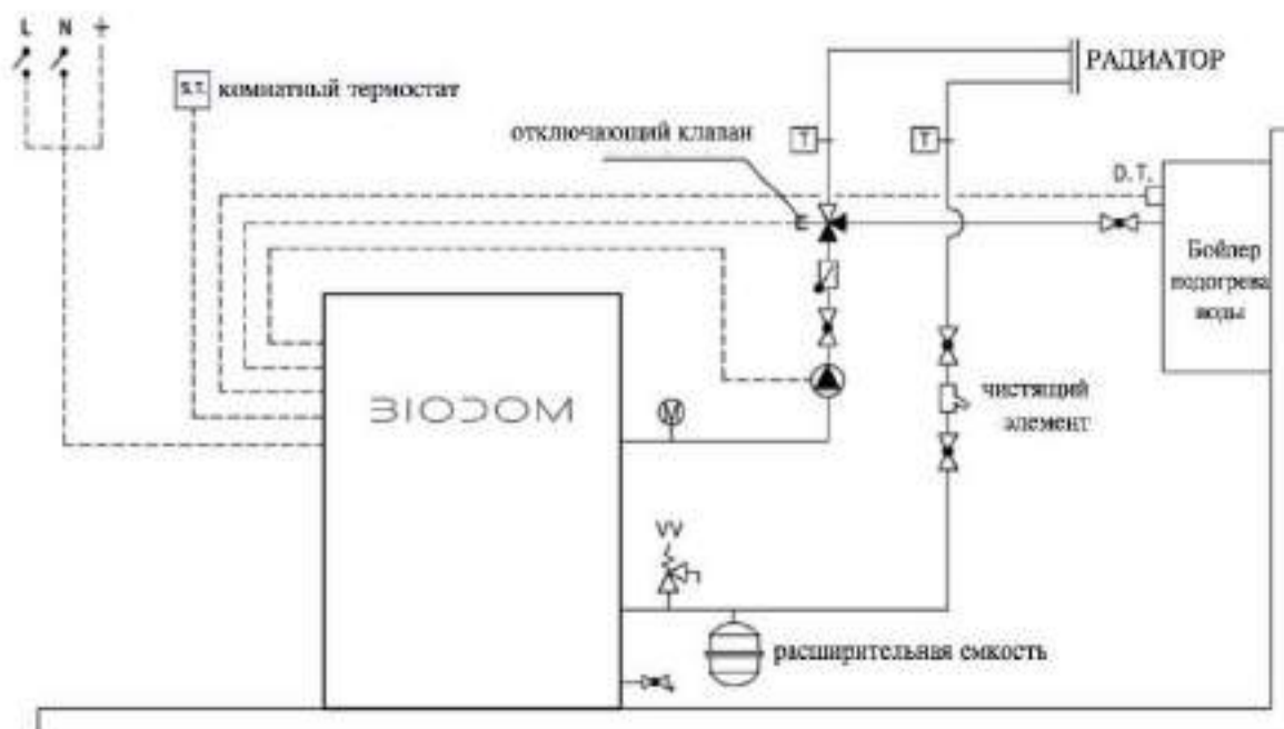
Схема подключения 2
