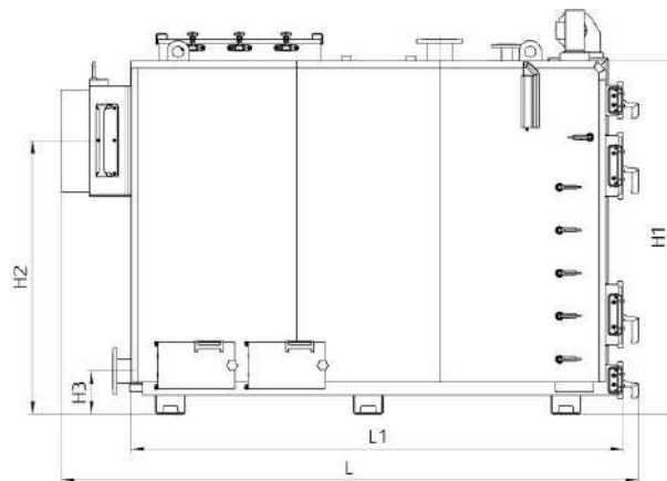
Рисунок 1 – Габаритный чертёж котла типа КТ-3Е
