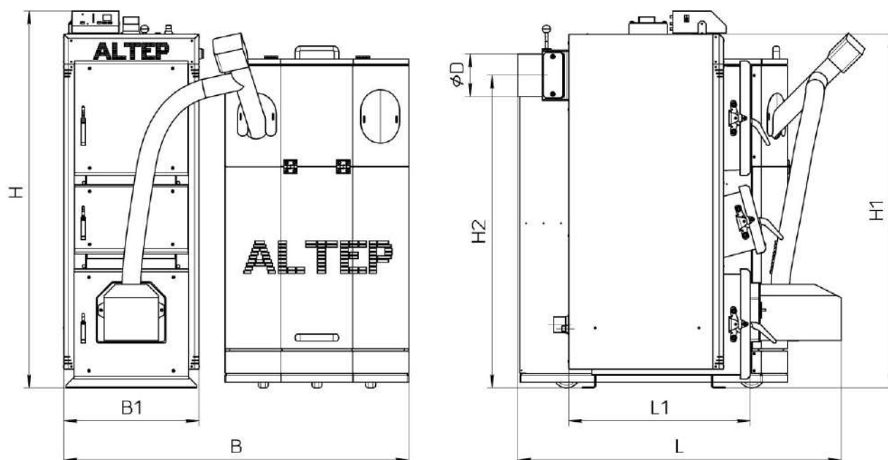
Рисунок 1 – Габаритный чертеж котла типа КТ-2Е-PG
